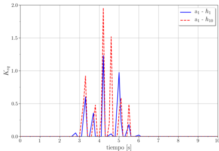
Figura 8. Evolución temporal del FIT equivalente para dos fisuras situadas en cotas distintas.
