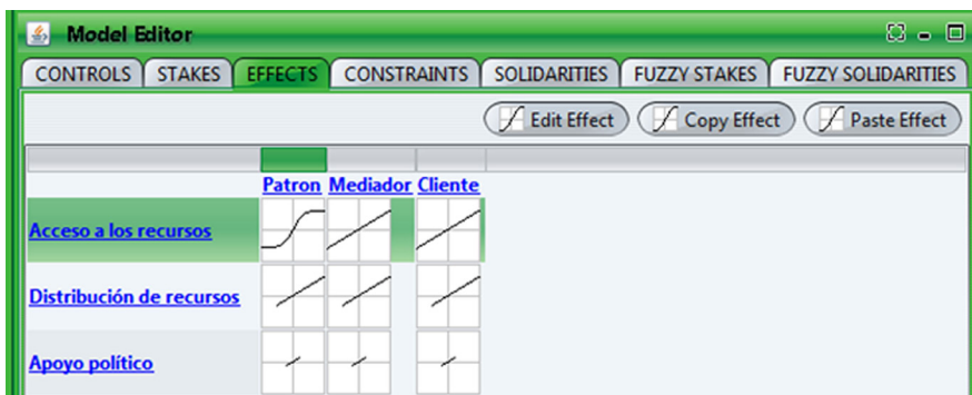
FIGURA 11 EDITOR DE PARÁMETROS. FUNCIONES DE EFECTO
