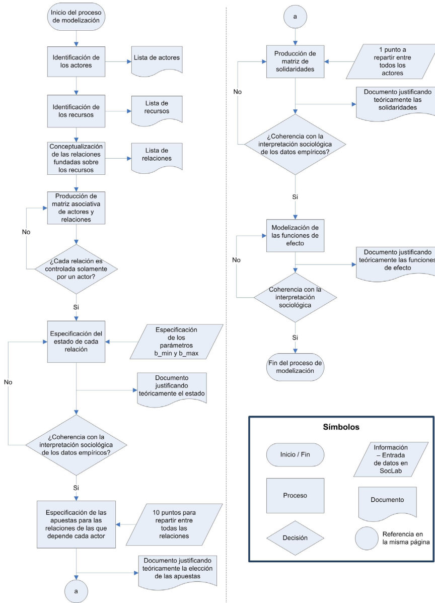
FIGURA 6 DIAGRAMA DE FLUJO DE LA METODOLOGÍA DE SocLAB
