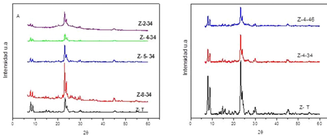
Figura 1. Patrones de DRX de las zeolitas (Z-T) y jerarquizadas. A) Efecto del tiempo de cristalización; B) Efecto de las relaciones molares CTAB/ SiO 2 en el gel de síntesis.
