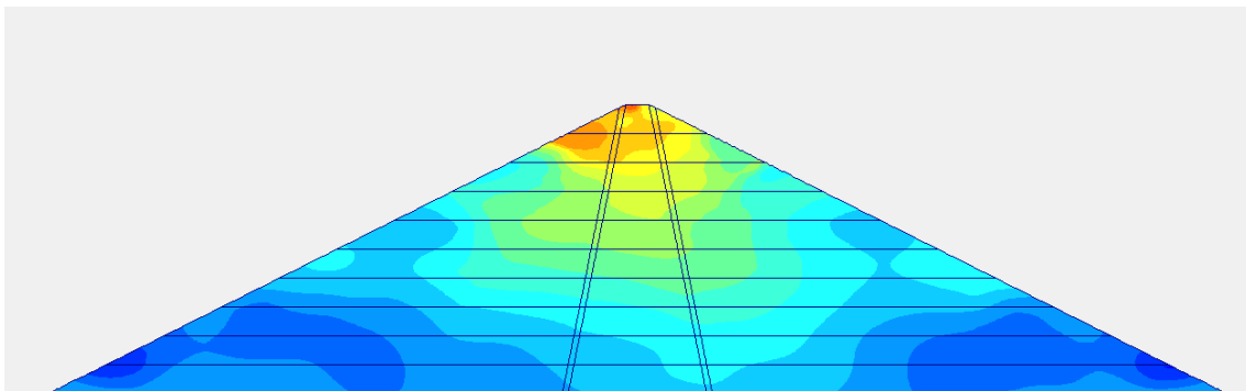
Fig. 6.14. Aceleraciones horizontales máximas registradas durante la simulación del sismo de Chi-Chi, Taiwán, CHY080-090.
