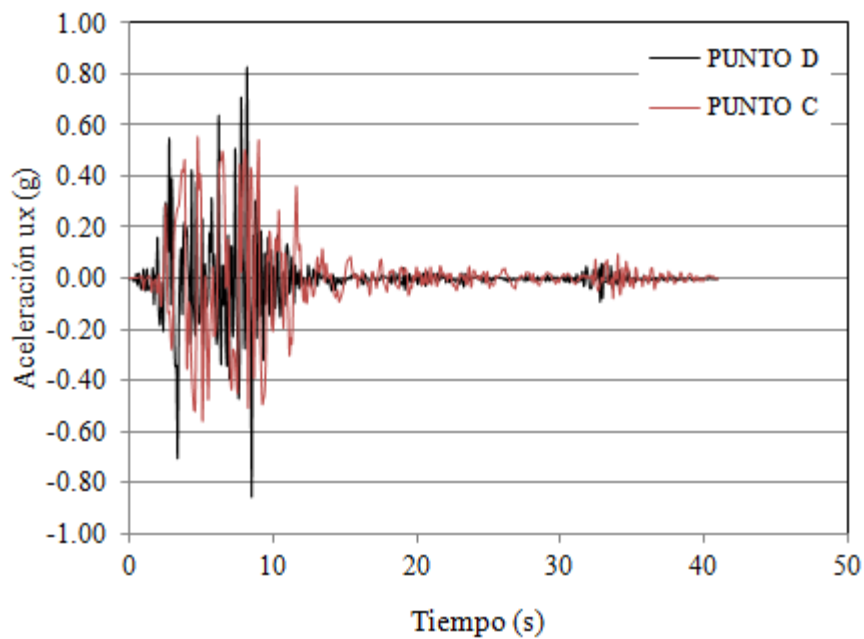
Fig. 6.11. Amplificación de las aceleraciones para el sismo de San Fernando, EEUU, desde la base de la presa hasta el coronamiento.
