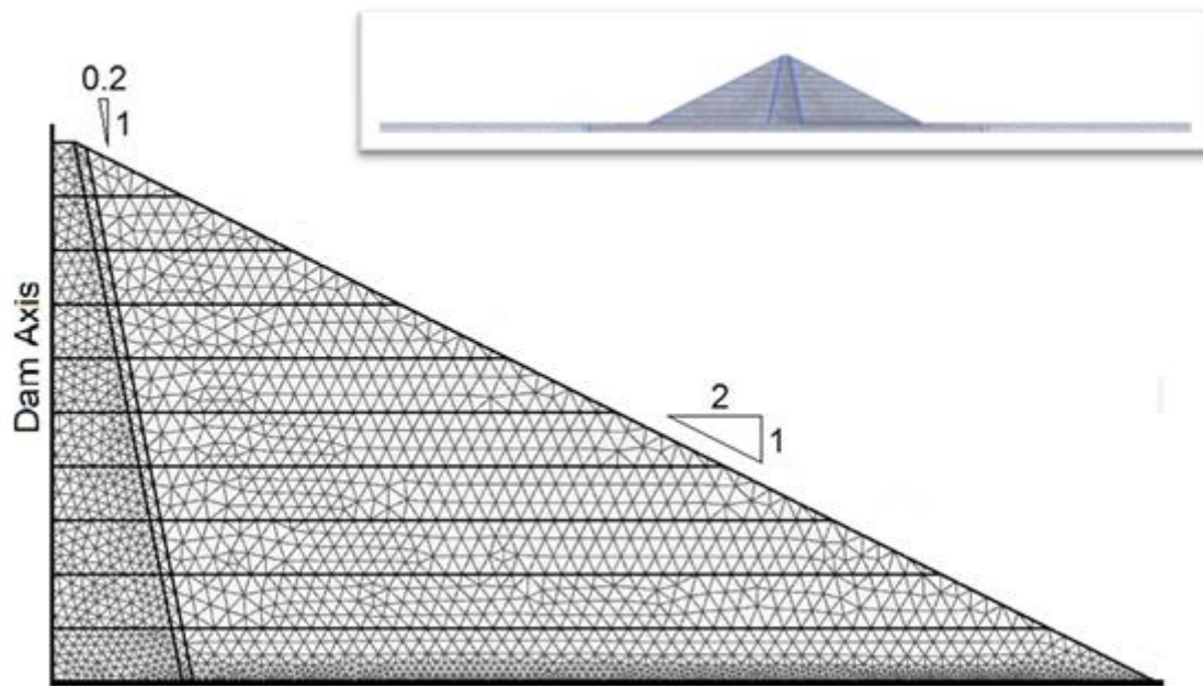
Fig. 6.5. Geometría del modelo y malla de Elementos Finitos
