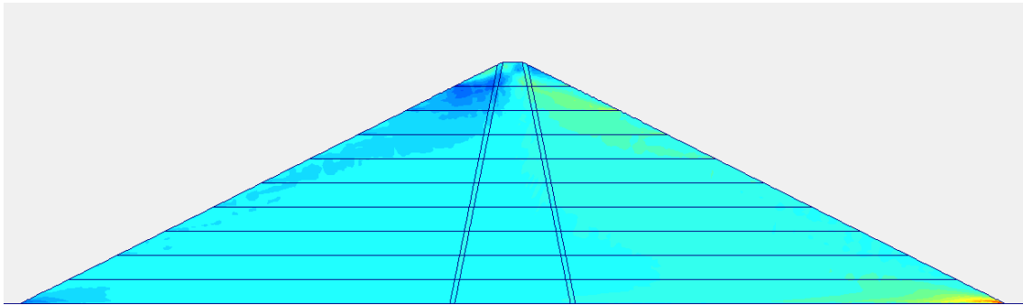
Fig. 6.13. Deformaciones cortantes resultantes de la simulación del sismo de Chi-Chi, Taiwán, CHY080-090.
