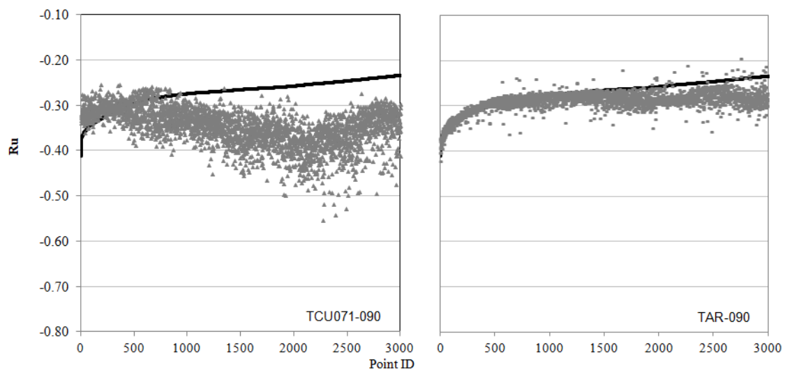
Fig. 6.12. Relación de presión de poros, para los sismos TCU071 y TAR-090. La línea llena representa la condición estática y los puntos los resultados post-sismo.
