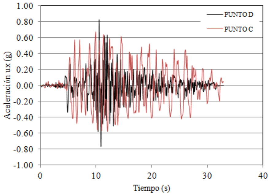
Fig. 6.10. Amplificación de las aceleraciones para el sismo de Tabas, Irán, desde la base de la presa hasta el coronamiento.
