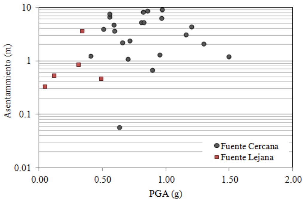
Fig. 6.9. Asentamientos del coronamiento obtenidos para el prototipo de 100 m con núcleo impermeable, sometidos a los sismos propuestos.
