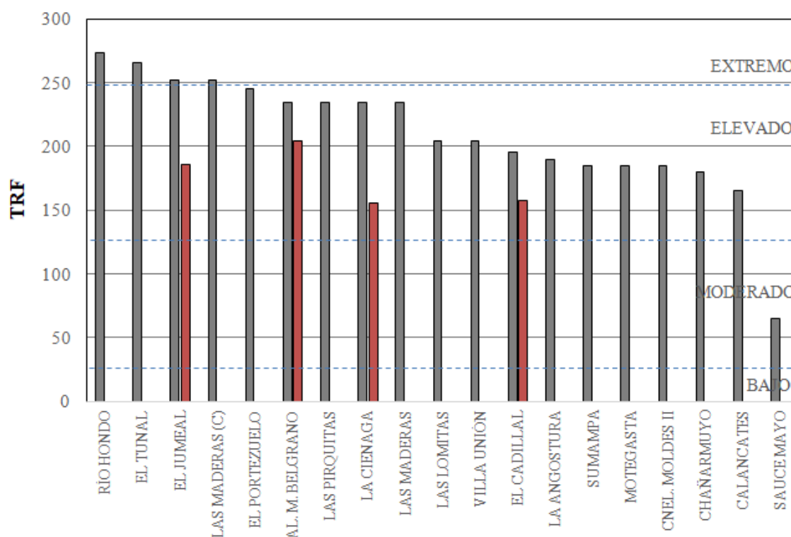
Fig. 5.2. Modificación del TRF para los casos analizados con el Ivsp.
