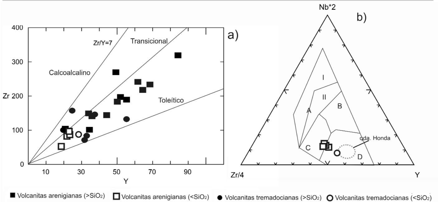
Figura 6: a) Relación Zr vs Y, donde es posible definir la filiación calcoalcilina y toleítica para las volcánitas analizadas (clasificación propuesta por Barrett y MacLean 1999). b) Diagrama triangular Zr/4 - Nb*2 - Y (Meschede 1986) para discriminar tectónicamente las rocas analizadas y compararlas con sus equivalentes básicos de la región de la Puna occidental.
