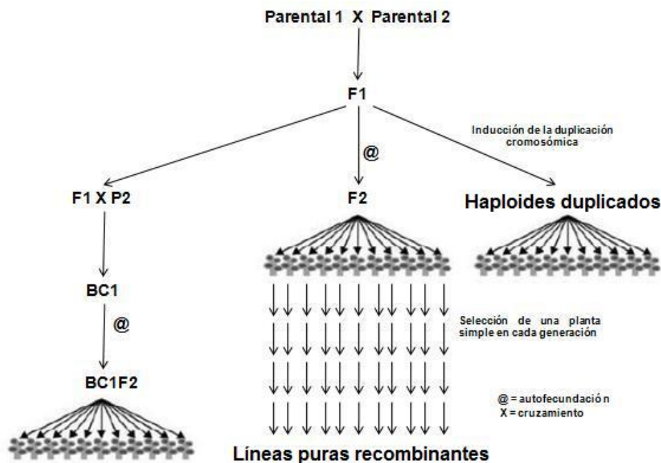
Figura 4. Diagrama de los principales tipos de poblaciones de mapeo (Collard et al., 2005).
