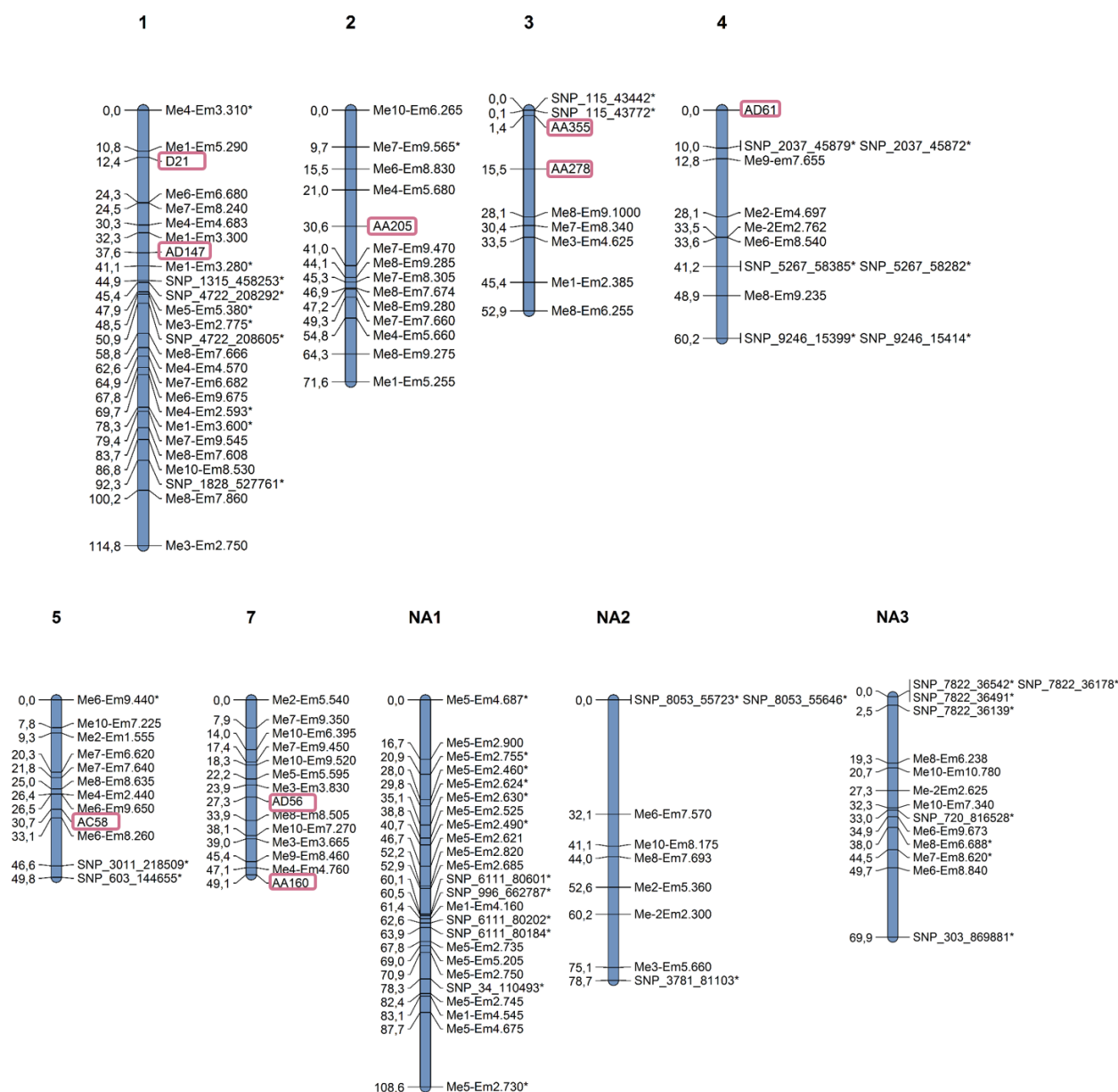
Figura 13. Mapa genético de Pisum sativum . El nombre de los marcadores se muestra a la derecha de cada grupo de ligamiento y las distancias en cM a la izquierda. Se indican con un asterisco los marcadores que presentaron segregación distorsionada ( 0,01 \leq p \leq 0,001 ). Los grupos de ligamiento fueron asignados en función a los marcadores SSR presentes en los mismos indicados con un recuadro rosa. NA corresponde a los grupos de ligamiento que no fueron alineados con el mapa de referencia.
