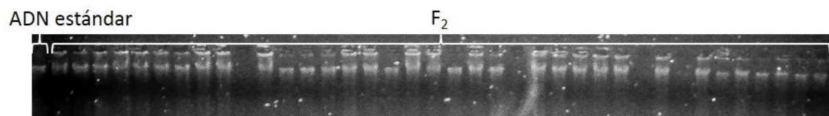
Figura 10. Gel de agarosa 1 %. Se observan extracciones de ADN genómico de los individuos de la población y el ADN estándar utilizado para cuantificar la cantidad de ADN (100ng/ \mu l).
