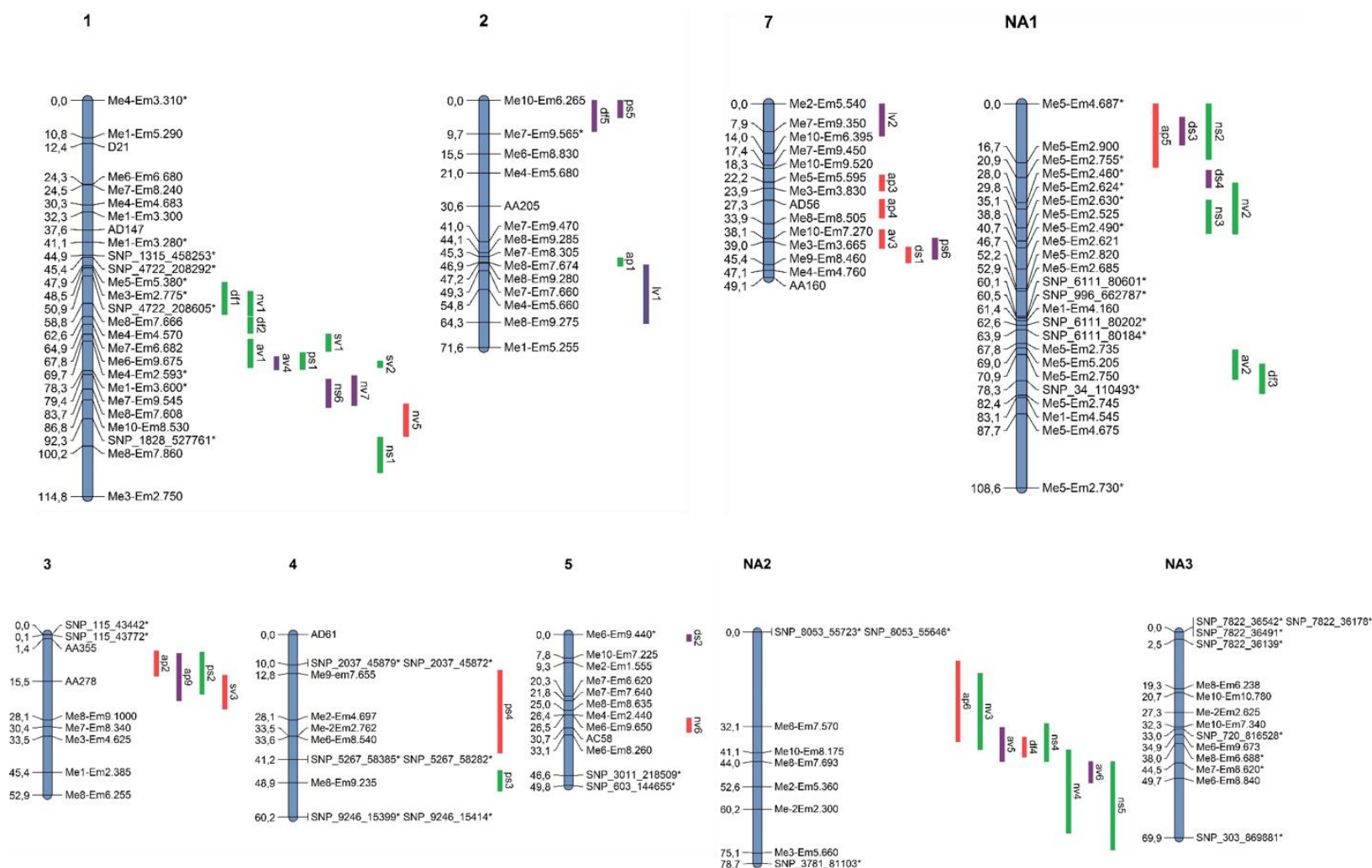
Figura 14. Posición de los QTLs asociados a los caracteres de interés en arveja detectados en la población derivada del cruzamiento de Explorer y DDR14 por el método CIM utilizando el mapa genético de Pisum Sativum generado a partir de los marcadores SSR, SRAP y SNP. Se indica con un asterisco los marcadores que presentaron segregación distorsionada ( 0,01 \leq p \leq 0,001 ). Se muestran los QTLs detectados en la población F 2 con color rosa, los detectados en la población F 2,3 evaluada en el 2014 con color verde y los de la población F 2,3 evaluada en el 2015 con color violeta.
