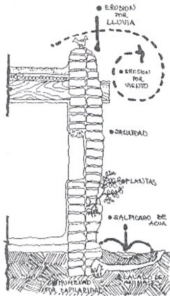
Factores que afectan a una construcción en tierra
