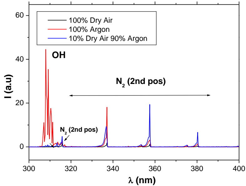
Figura 14. Bandas de emisión vibro rotacionales del OH y el N 2 , de un plasma de descarga de gases operado en aire seco 1 L/min (línea negra), Ar 1 L/min (línea roja) y 10% aire seco más 90% Ar (línea azul). Barrido entre los 300 y 400 nm utilizando el fototubo visible.
