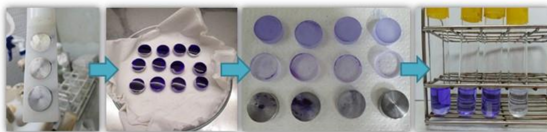
Figura 3. Secuencia del procesamiento de los cupones para la evaluación indirecta de la formación de biofilm de P. aeruginosa en tres superficies abióticas. De arriba hacia abajo en la figura: policarbonato, vidrio y acero inoxidable.
