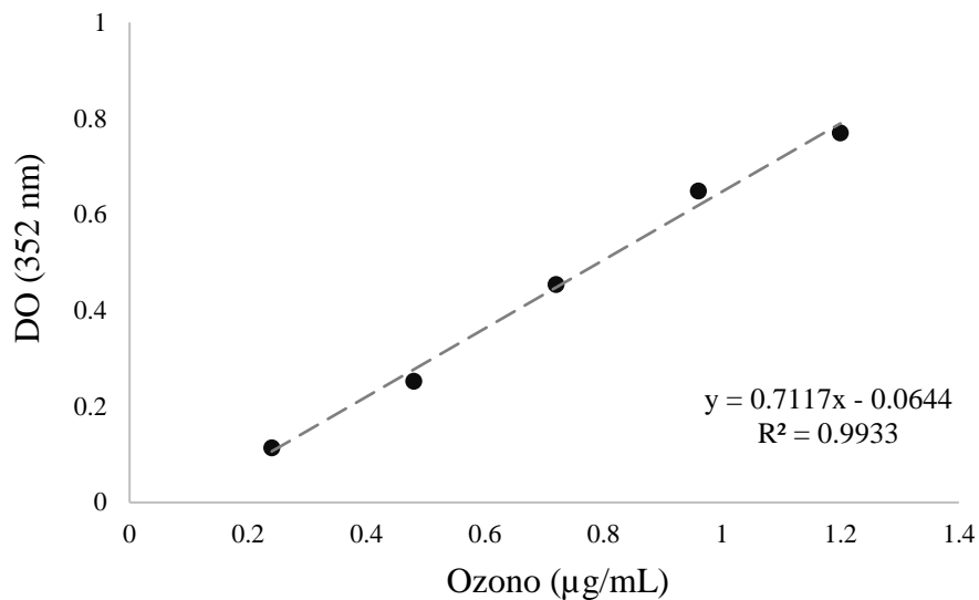
Figura 23. Curva de calibración densidad óptica a 352 nm ( \text{DO}_{352} ) a diferentes concentraciones de ozono ( \mu\text{g/mL} )
