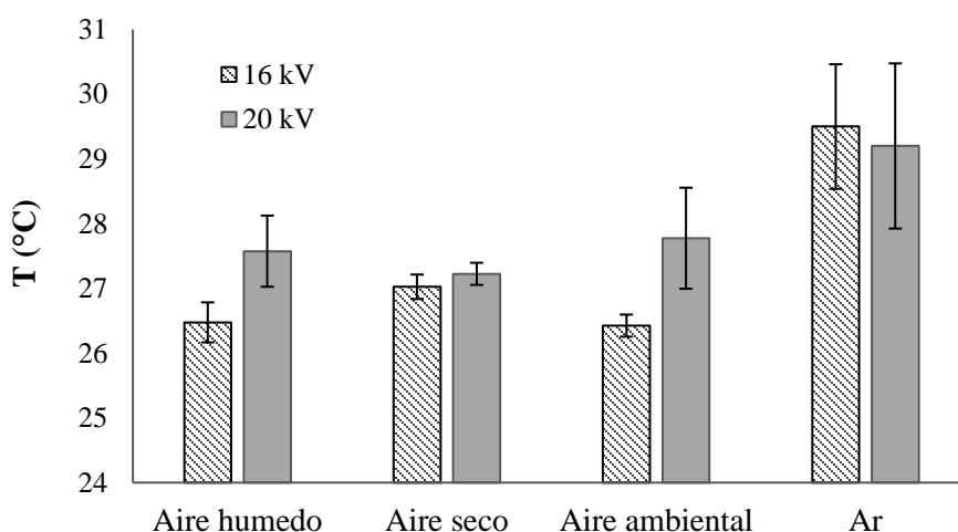
Figura 22. Temperaturas obtenidas con una cámara infrarroja del gas efluente del plasma operado en aire humedecido, seco y ambiental y en Ar, utilizando un voltaje de 16 y 20 kV. Las barras representan la desviación estándar.
