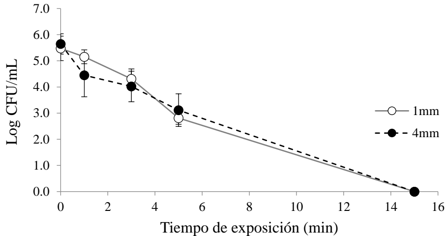
Figura 7. Curva de supervivencia de biofilm de P. aeruginosa tratado con dispositivo DBD de plasma en aire ambiental circundante durante diferentes tiempos de exposición. Fuente de plasma localizada a 1 o 4 mm de la superficie de la muestra (línea continua y punteada, respectivamente). Las barras de error representan el error estándar de la media. Los resultados son el promedio de 4 experimentos independientes, cada uno por duplicado.
