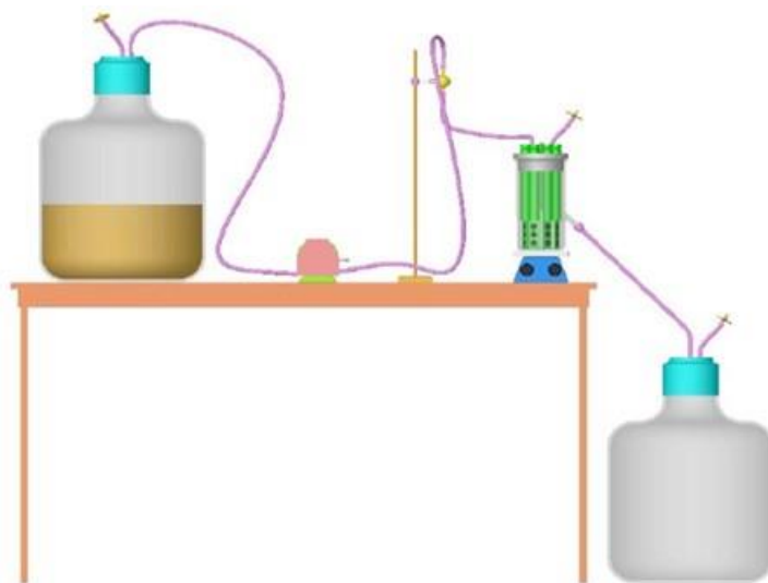
Figura 2. Esquema del sistema continuo para el crecimiento del biofilm de P. aeruginosa (CDC Biofilm Reactor Operator Manual, Biosurface Technologies Corp., 2003)
