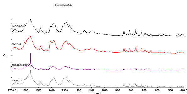
Fig.12: Espectro FTIR de tejidos de Algodón, Modal, Microfibra y Anti-UV rango “huella dactilar” 1700 a 400 \text{cm}^{-1}
