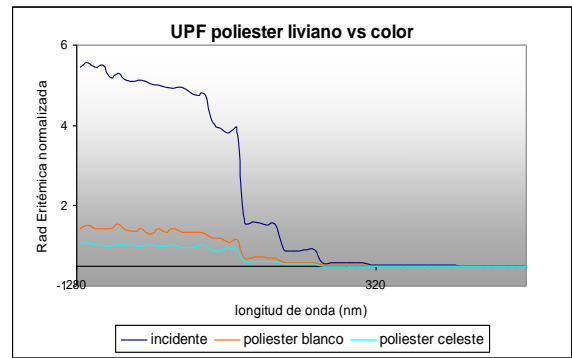
Fig.9: Transmittancia eritémica para poliéster liviano de distinto color
