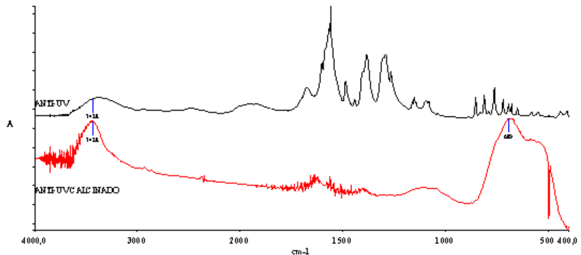
Fig. 16: FTIR de tejido de Anti-UV y residuo calcinado a 700°C
