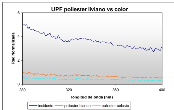
Fig.8: Transmittancia para poliéster liviano de distinto color
