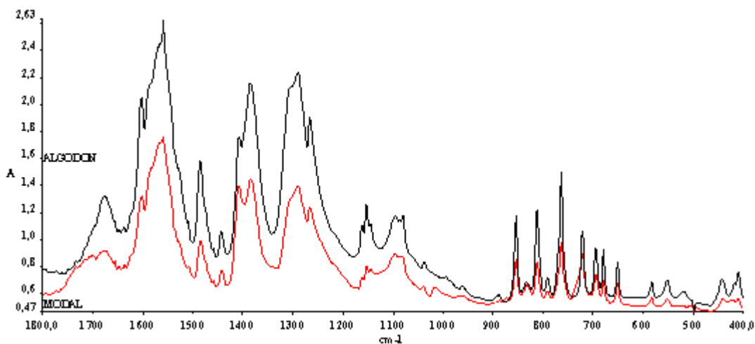
Fig.13: Espectros FTIR de Algodón y Modal en la región de la “huella dactilar”
