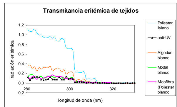
Fig.3: Espectros de radiación eritémica incidente / transmitida
