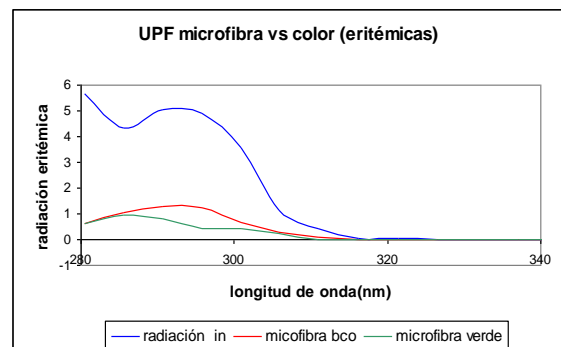
Fig.5: Transmitancia eritémica para microfibra de distinto color
