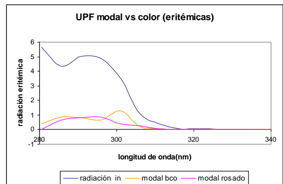
Fig.7: Transmitancia eritémica para modal de distinto color
