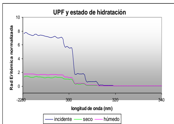
Fig.10: Transmittancia eritémica para poliéster liviano de distinto estado de hidratación.
