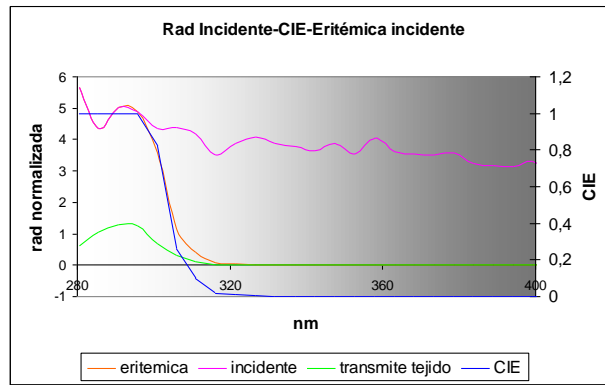
Fig. 1: Irradiancia incidente normalizada, irradiancia eritémica incidente, espectro CIE e Irradiancia eritémica transmitida por un tejido en nuestro espectrómetro.
