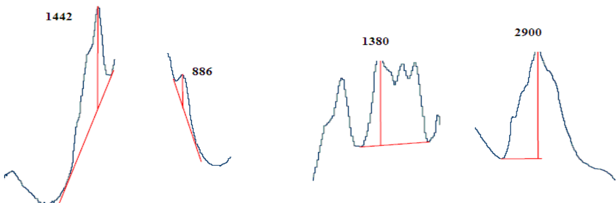
Fig.14: Índice de cristalinidad Total a partir de la altura media de las absorbancias
