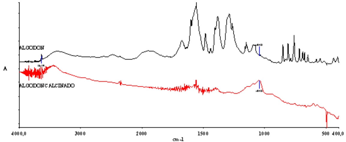
Figura 15: FTIR de tejido de Algodón y residuo calcinado a 700°C
