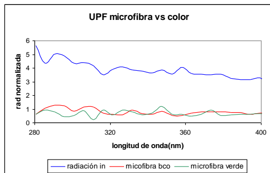
Fig.4: Transmitancia para microfibra de distinto color
