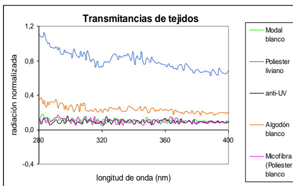
Fig.2: Espectros de radiación incidente / transmitida
