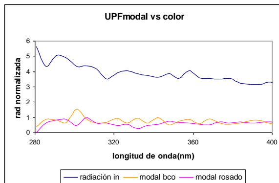
Fig.6: Transmitancia para modal de distinto color
