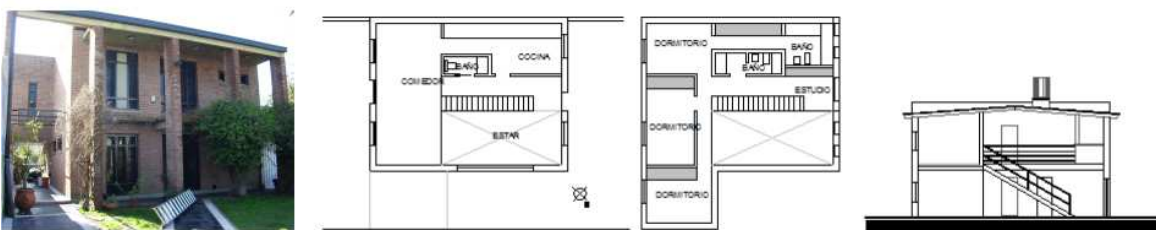
Fig. 3: Fachada plantas y corte de la vivienda.
