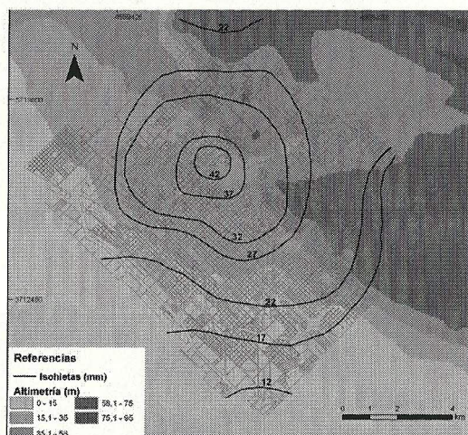
Fig. 5. Distribución de los valores de precipitación del 18 de diciembre de 2008 en la ciudad de Bahía Blanca.
