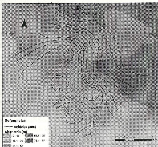
Fig. 4. Distribución de los valores de precipitación del 24 de noviembre de 2008 en la ciudad de Bahía Blanca.
