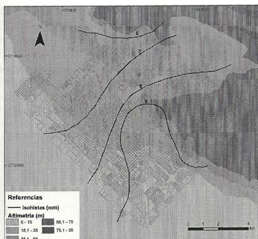
Fig. 3. Distribución de los valores de precipitación del 10 de mayo de 2009 en la ciudad de Bahía Blanca.
