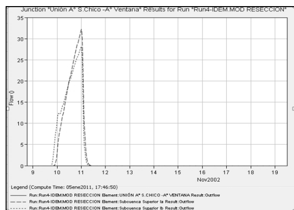
Figura 9. Evento Nov/2002 - Hidrogramas de las Subcuencas Ia y Ib en el punto de unión (Balneario Tornquist).
