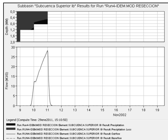
Figura 8. Evento Nov/2002 - Hidrograma en Subcuenca Superior Ib.
