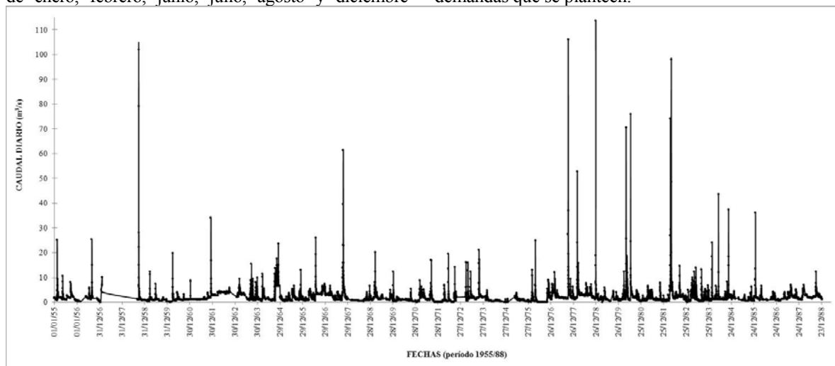
Figura 2. Río Sauce Chico – Estación HL6005-ADA- Serie histórica de caudales diarios – Período 1955/88: 10587 datos.
