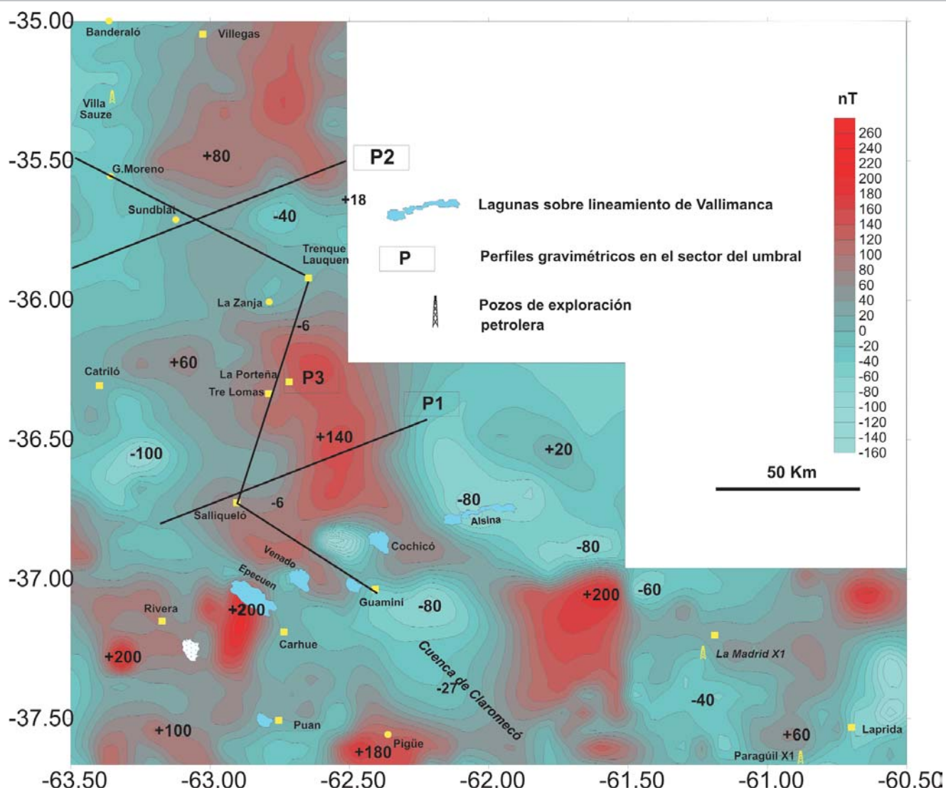
Figura 4: Mapa de de anomalías del campo magnético terrestre. Isolinías cada 20 nanoTeslas.
