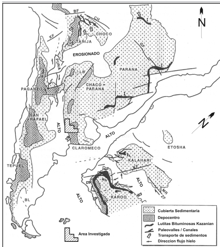
Figura 1: Mapa con la ubicación de los depocentros paleozoicos (modificada de Tankard et al. 1995).
