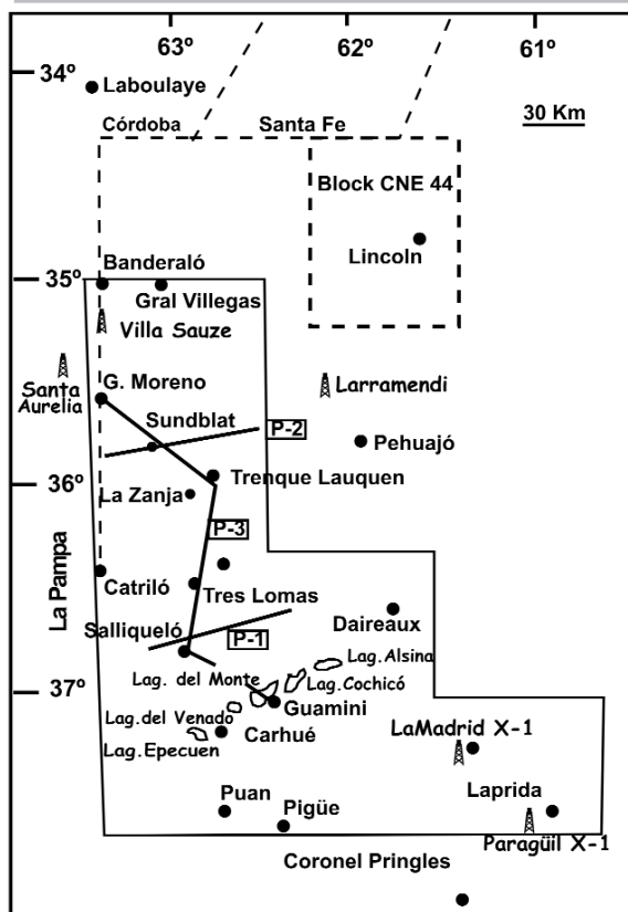
Figura 1: Mapa con la ubicación de los depocentros paleozoicos (modificada de Tankard et al. 1995).
