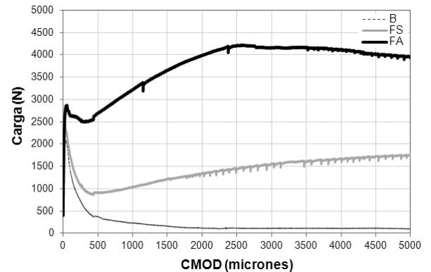
Figura 10. Curvas Carga-CMOD.
