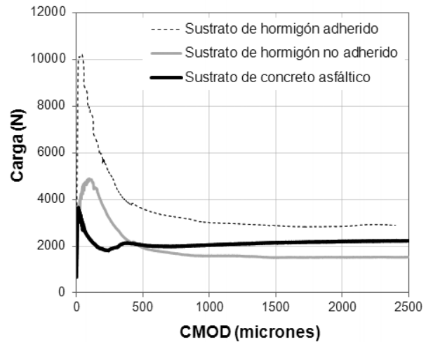
Figura 8. Experiencias preliminares Izquierda: Respuesta en flexión de probetas compuestas sobre un sustrato de hormigón simple reforzadas con un overlay de hormigón simple y con el mismo overlay reforzado con 40 kg/m 3 de fibras de acero tipo hooked end. Derecha: Curvas carga – COD de overlay con 3,5 kg/m 3 de macrofibras sintéticas aplicados sobre distintos sustratos
