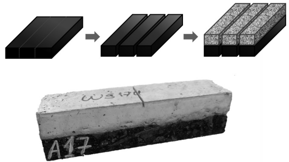
Figura 4. Proceso de elaboración de las vigas compuestas.
