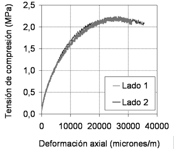
Figura 7. Ensayo de compresión sobre el sustrato de concreto asfáltico.
