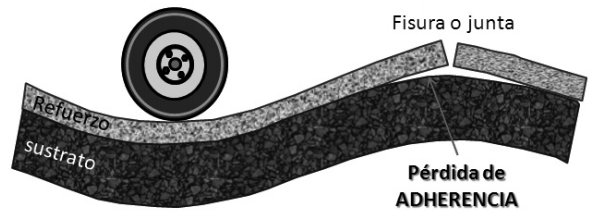
Figura 2. Efecto del tránsito sobre el compuesto.
