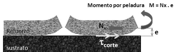
Figura 3. Solicitaciones que causan la pérdida de adherencia
