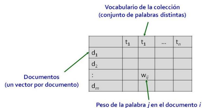
Figura 3. Representación vectorial de los documentos
