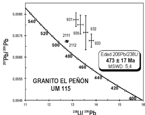
FIG. 6. Diagrama U-Pb Tera-Wasserburg para circones del Granito El Peñón. (931, 2111, etc., corresponden al número de laboratorio de las fracciones analizadas).
