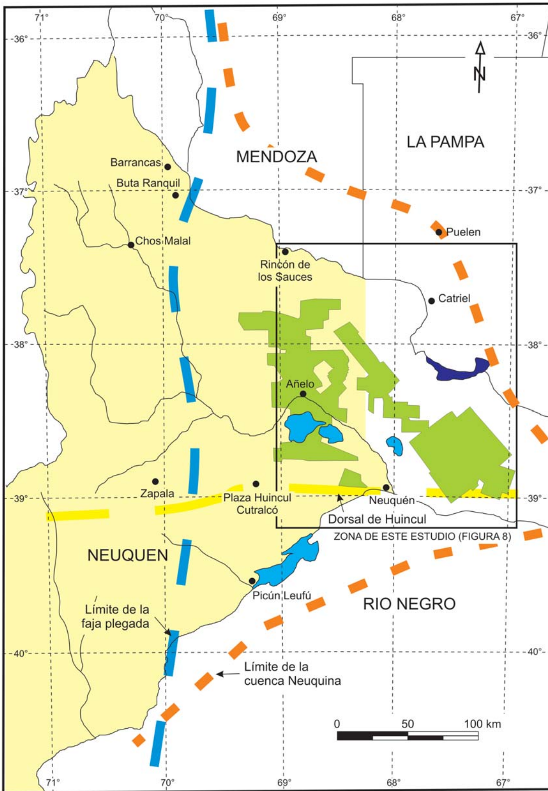
Figura 1: Ubicación de la región de estudio. Se muestra también, en color verde, la cobertura de sísmica 3D utilizada para este trabajo.
