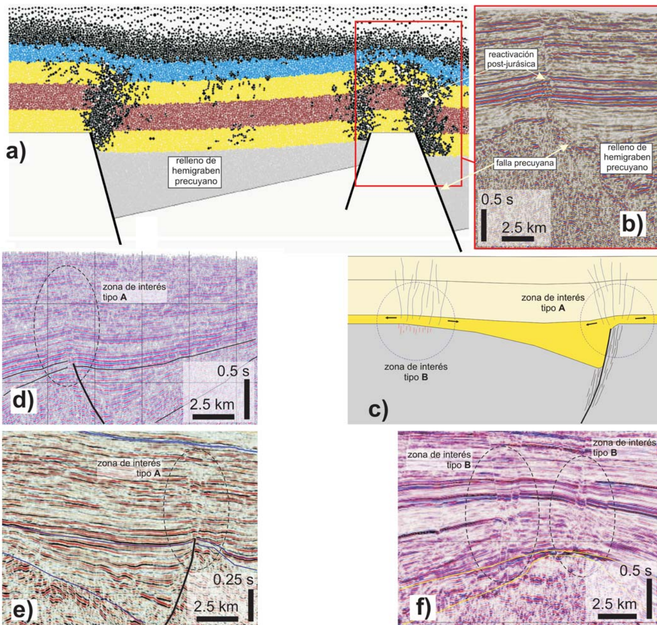
Figura 9: a) Simulación numérica por elementos discretos del mecanismo de subsidencia diferencial. En negro se pintaron los elementos que soportaron la tensión por estiramiento de las capas (tomado de Cristallini et al. 2006); b) Sección sísmica de Entre Lomas comparando con el modelo; c) Esquema donde se indican las zonas de tensión que tienen interés económico ya que son sectores donde se genera espacio por fracturamiento; d, e y f) Ejemplos de la región de Bandurria- Loma La Lata.
