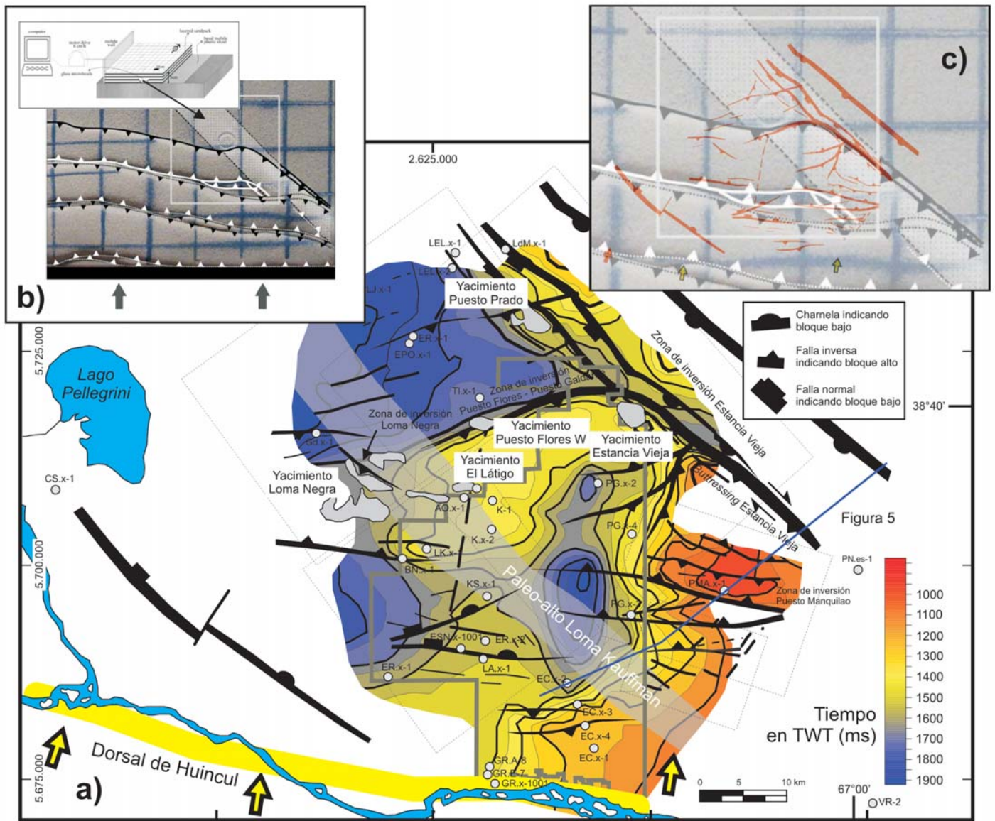
Figura 4: a) Mapa de la estructura jurásica superior en la región de Estancia Vieja-Loma Kaufman donde se indican las principales fallas de la región. Se muestra también el isócrono de la base del Grupo Cuyo que resalta el plegamiento resultante y la posición del alto precuyano de Kauffman para correlacionar con el mapa de la figura 3. En línea punteada se indica la cobertura de sismica 3D; b) Modelo análogo tomado de Yagupsky et al. (2008) donde se muestra la inversión selectiva sobre un hemigraben oblicuo. Se indica blanqueada la posición de un hemigraben por debajo del modelo; c) Comparación del modelo con la estructura de Estancia Vieja y Puesto Flores-Puesto Galdame.
