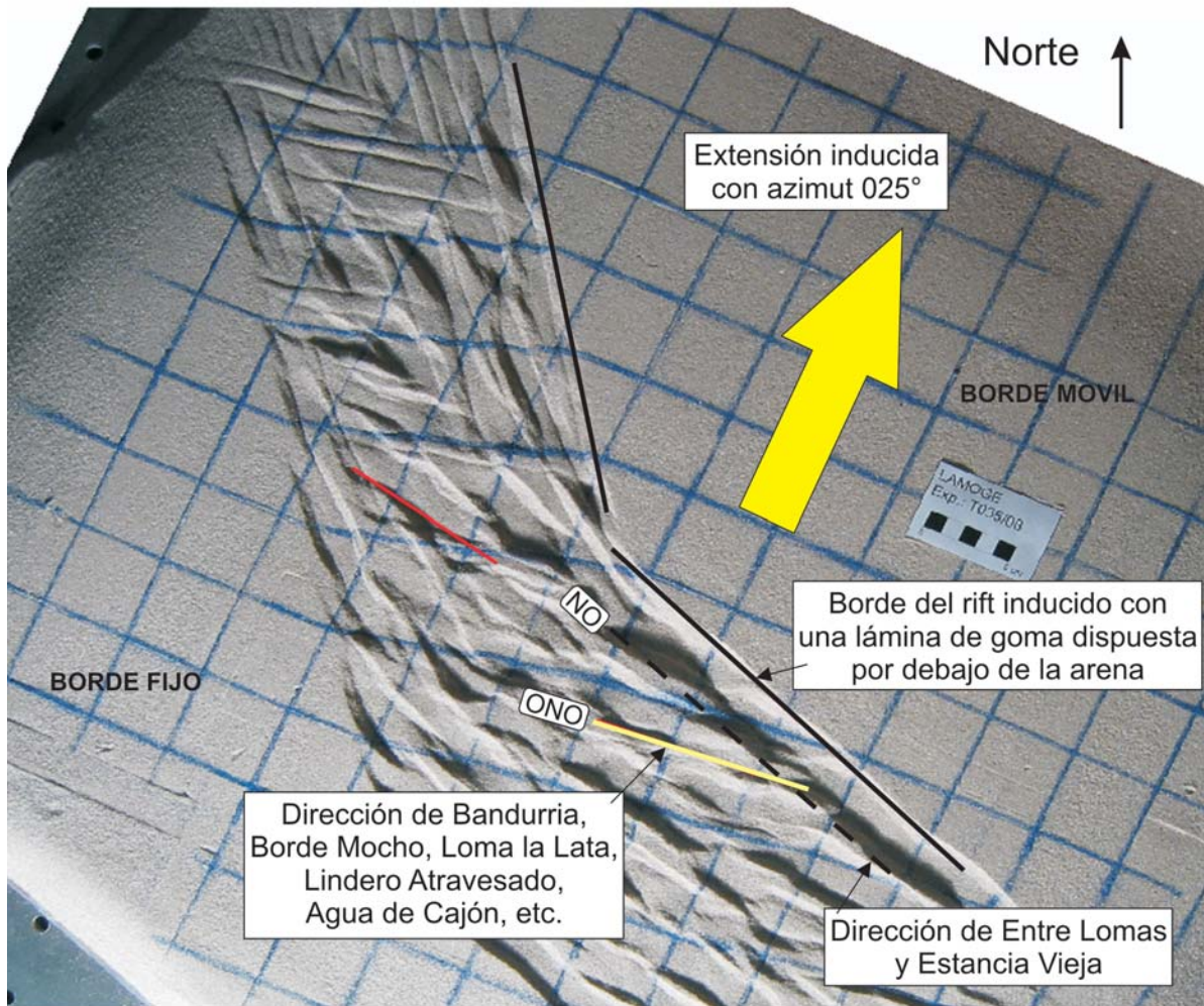
Figura 11: Modelo análogo de rift oblicuo realizado por Bechis (2009) que permite explicar las dos direcciones de estructuras precuyanas. El borde del rift está dispuesto oblicuamente a la dirección de extensión. Los sistemas de fallas noroeste (Entre Lomas, Estancia Vieja) serían paralelos al borde del rift, mientras que los de orientación este-noroeste serían ortogonales a la dirección de extensión.
