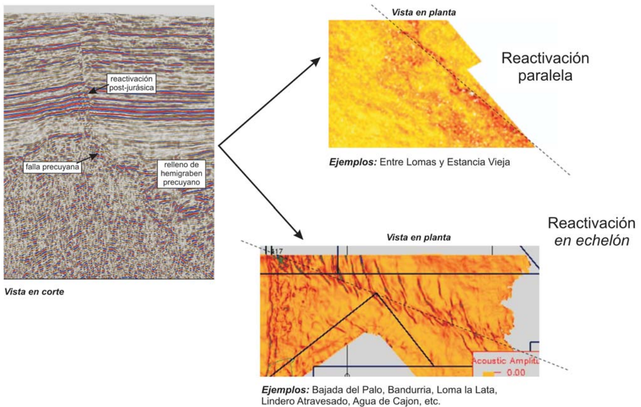
Figura 10: Las reactivaciones jurásico-cretácicas se pueden dividir en dos grupos. Uno de ellos (reactivación tipo Entre Lomas o paralela) en que las fallas normales jurásico-cretácicas se desarrollan paralelas a las estructuras precuyanas de orientación noroeste. El otro grupo corresponde a las reactivaciones tipo Bandurria (o en echelón) en que las fallas jurásico-cretácicas se disponen en echelón sobre las precuyanas que tienen dirección oeste-noroeste. Las vistas en planta corresponden al atributo de inclinación (dip) del reflector base de la Formación Vaca Muerta.
