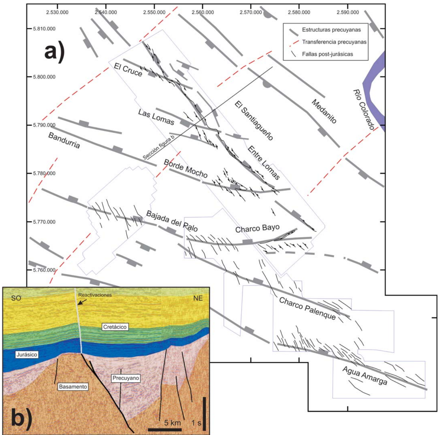
Figura 6: a) Mapa de la región de Entre Lomas donde se muestran las principales fallas y zonas de transferencia precuycanas (en gris) y las fallas normales jurásico-cretácicas (en negro). Nótese la interferencia entre los patrones precuycanos noroeste y oeste-noroeste; b) Sección sísmica representativa de la estructura de Entre Lomas y hemigraben El Santiagueño.
