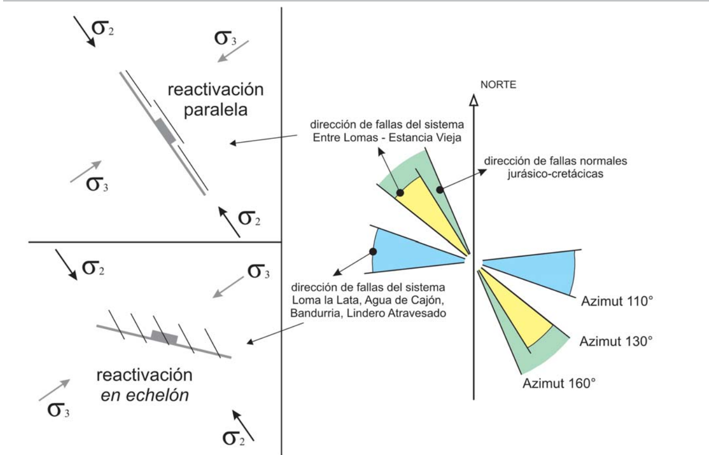
Figura 12: Distribución de esfuerzos compatibles con las estructuras jurásico-cretácicas y comparación con las direcciones estructurales precuyanas. Esta situación implica una rotación horaria del esfuerzo principal mínimo ( \sigma_3 ) desde una orientación nor-noreste en el Triásico Superior - Jurásico Inferior a una dirección noreste en el Jurásico Superior-Cretácico Inferior.
