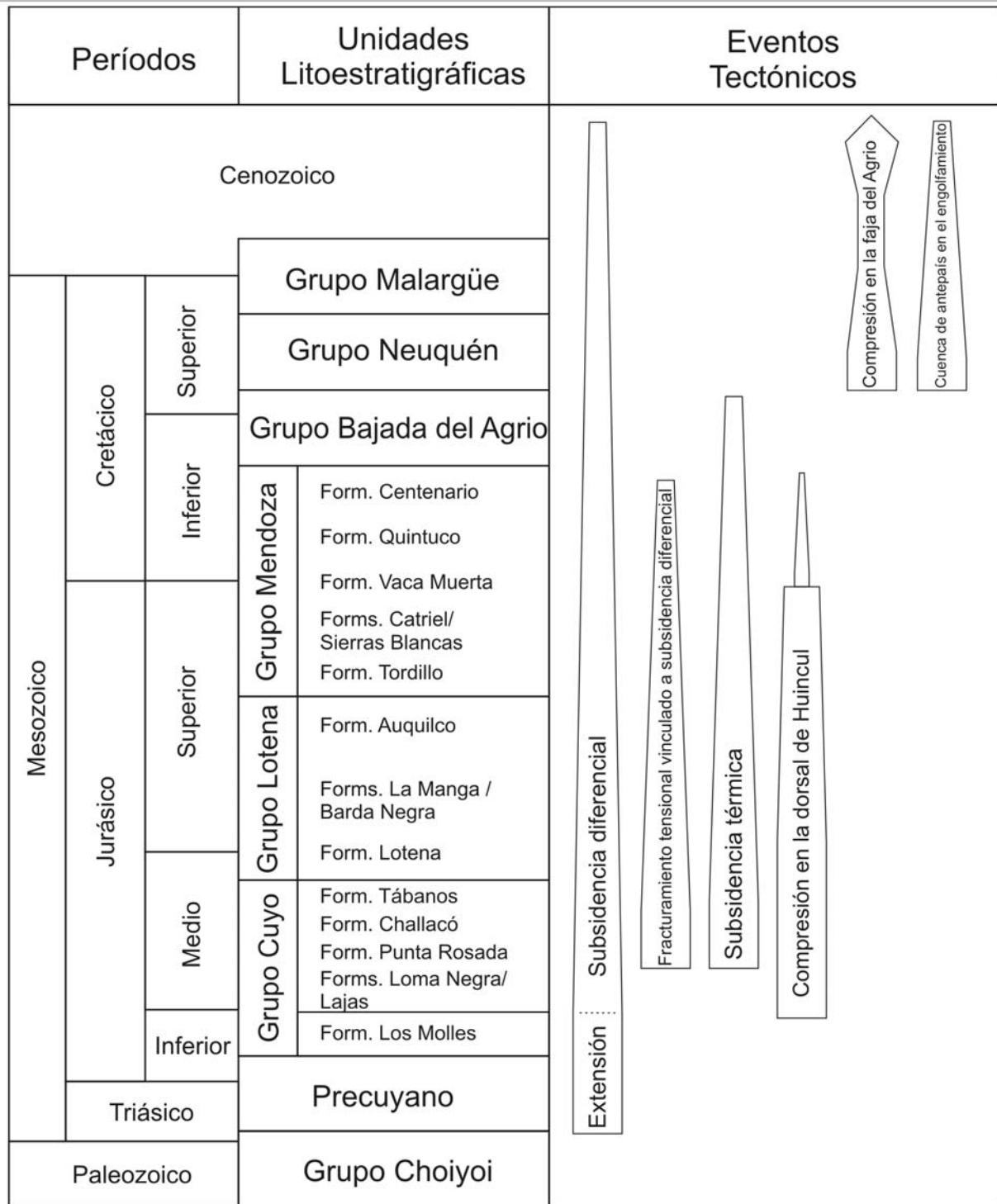
Figura 2: Cuadro tectonoestratigráfico donde se muestran las principales unidades y procesos mencionados en el texto.
