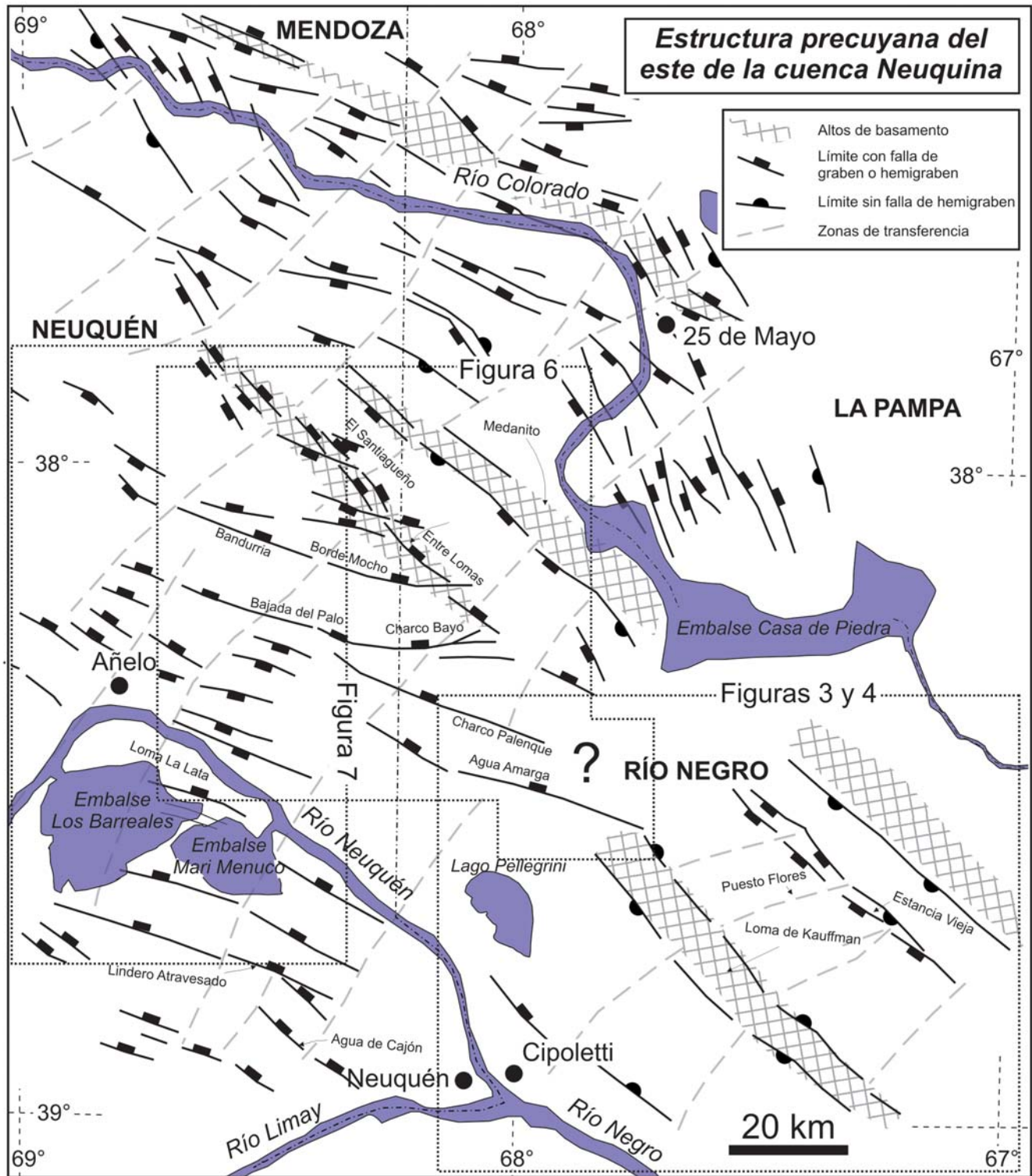
Figura 8: Principales fallas y transferencias desarrolladas durante el Triásico Superior - Jurásico Inferior en el este de la cuenca Neuquina. La dirección general de las fallas normales encontradas es noroeste. Sin embargo, existen dos poblaciones bien marcadas. La primera de ellas (población noroeste) está compuesta por fallas con direcciones azimutales superiores a 130° (ej. fallas de los lineamientos de Entre Lomas y Estancia Vieja), la segunda (población oeste-noroeste) está compuesta por estructuras con direcciones azimutales inferiores a los 110° (ej. hemigrábenes de las zonas de Loma La Lata, Agua de Cajón, Lindero Atravesado, Bandurria, etc.).
