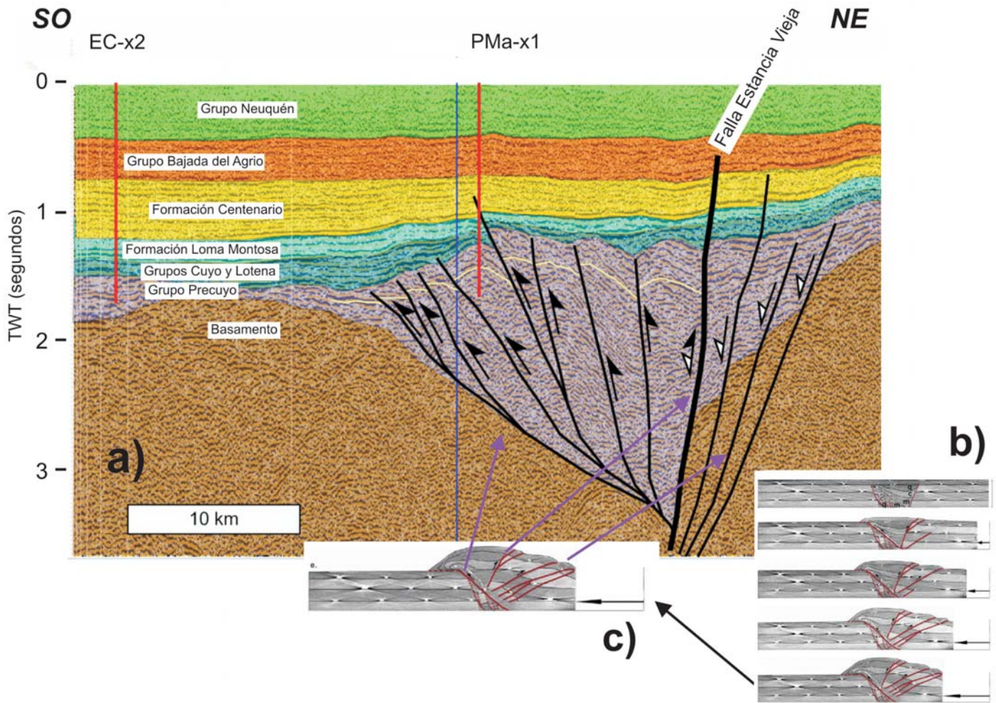
Figura 5: a) Sección sísmica en la que se muestran fallas inversas de orientación este-oeste, desarrolladas dentro de los hemigrábenes. Estas fallas en muchos casos están despegadas hacia la base del precuyano y están comprimiendo el relleno de los hemigrábenes contra la falla principal de Estancia Vieja (efecto de buttressing); b y c) Comparación de la información sísmica con un modelo análogo de Panien et al. (2005) donde se observa el efecto de extrusión del relleno del hemigraben a partir de fallas despegadas en la base del hemigraben. En el caso de la estructura analizada, estas fallas inversas no serían paralelas al hemigraben ya que la compresión es oblicua (en relación a la estructura extensional).
