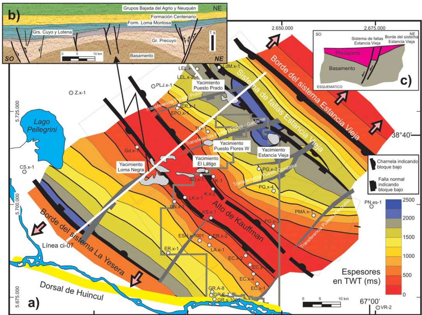
Figura 3: a) Mapa de las estructuras precuyanas en la región de Estancia Vieja-Loma Kaufman. Se se indican las principales fallas, zonas de transferencia y zonas de bisagra (hinges) de los hemigrábenes. Se muestra también, la tendencia de variación de espesores del precuyano; b) Sección sísmica 2D ci-07 que atraviesa los hemigrábenes de Estancia Vieja y La Yesera y el alto de Kaufman; c) Esquema mostrando la estructura de la cubeta de Estancia Vieja.
