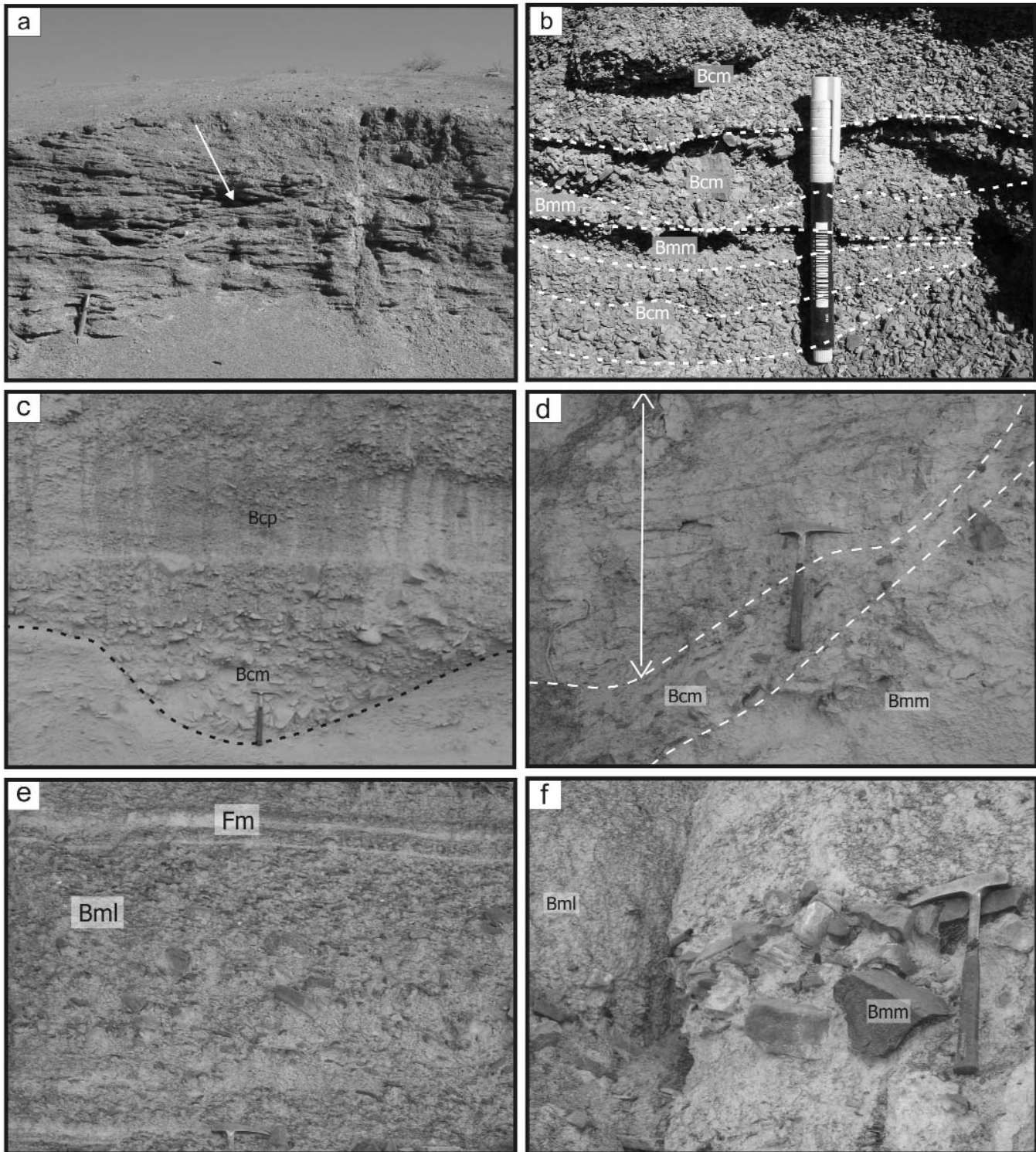
Figura 9: a) Vista general depósitos correspondientes a un abanico coluvial dominado por flujos fluidos, la flecha indica una de las superficies erosivas, b) Litofacies Bmm y Bem de la asociación de facies de abanicos coluviales dominados por flujos fluidos, e) Litofacies Bcm y Bcp de la asociación de facies de sistemas de río colector-conoide, d) Litofacies de canal y de abandono de canal (flecha) en depósitos de sistemas río colector-conoide, e) Litofacies Bml y Bmm en depósitos de sistemas río colector-conoide, f) Litofacies Bml y Fm en depósitos de sistemas río colector-conoide
