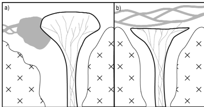
Figura 12: Relación entre el sistema río colector-conoide y el de transferencia. Estudios de progradación (A) y erosión (B).
