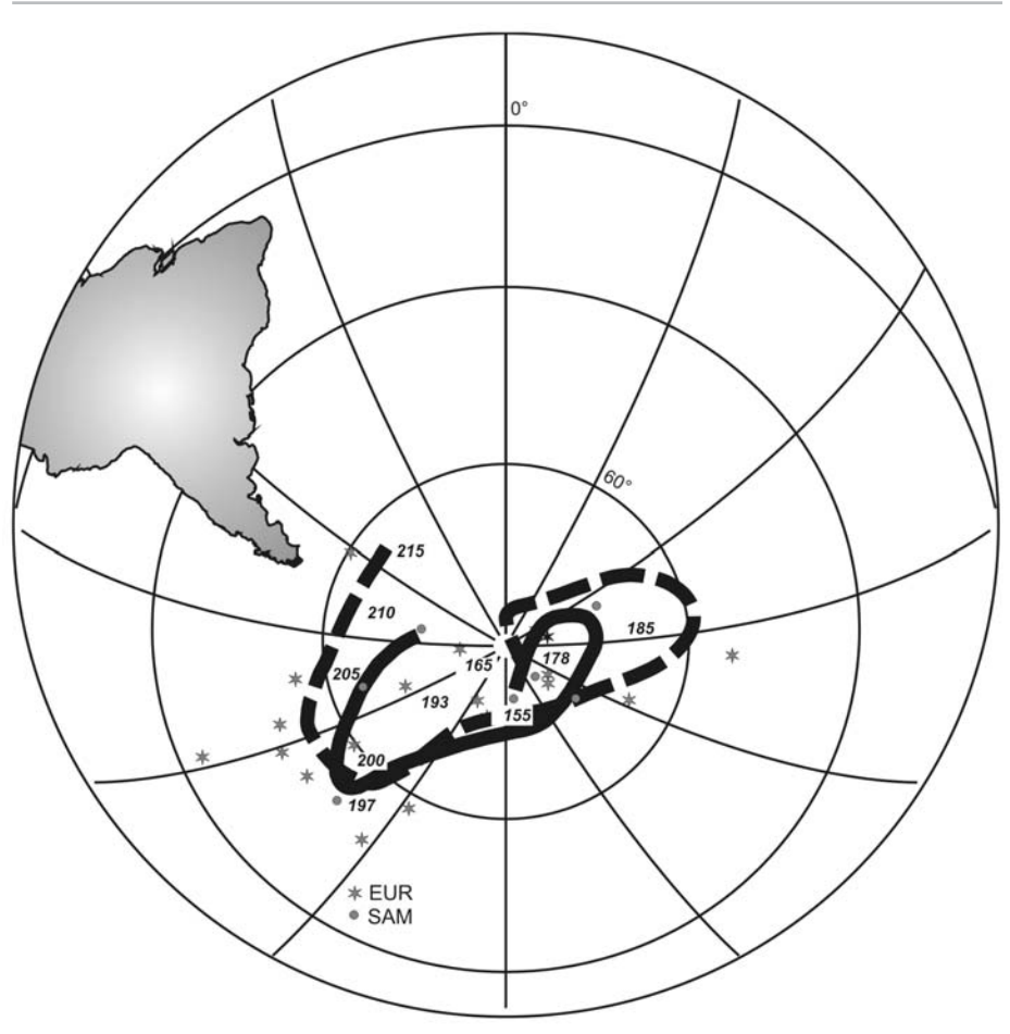
Figura 7: Curva de deriva polar aparente (CDPA) de América del Sur (línea llena) propuesta para el intervalo Triásico Tardío - Jurásico Tardío. La CDPA de Eurasia (línea entrecortada) construida con polos de la base de datos de Torsvik et al. (2001), resulta muy similar a la de América del Sur. Los PP de Eurasia fueron rotados a coordenadas de América del Sur usando dos modelos conocidos para Pangea, que varían para los dos grupos de edades bien definidos. La curva sugiere una deriva polar aparente y/o verdadera importante durante el Jurásico Temprano. Modelo 1 (para 220-193 Ma): EU-NA por Srivastava y Tapscott (1986), NA-SAF por Klitgord y Schouten (1986), SAF-SAM por Rabinowitz y La Brecque (1979), Modelo 2 (para 183-165 Ma), EU-NA, NA-AF y AF-SAM por Lawver y Scotese (1987). 210-155: edades reasignadas según Ogg (2004).
