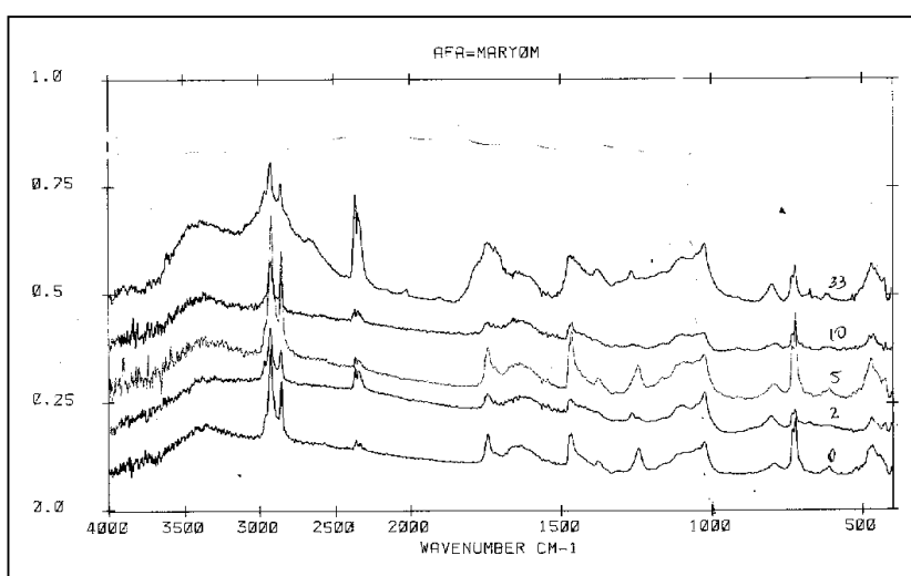
figura 6: espectro FTIR
