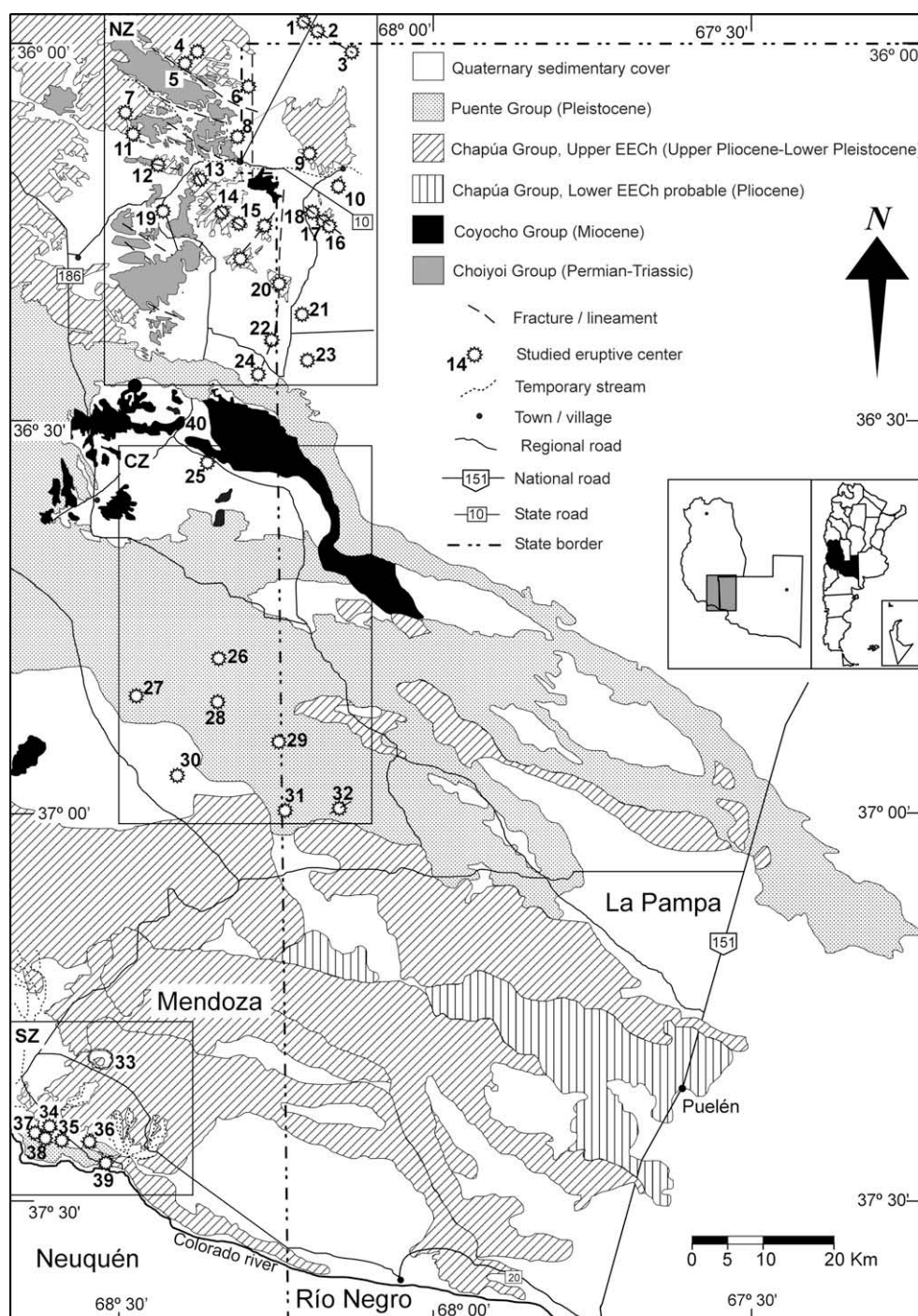
Fig. 2. Geological map of study area and volcanoes sampled (modified from Bertotto, 2003). Northern Zone (NZ): 1, Loma Chica Oeste; 2, Loma Chica Este; 3, Loma Chica Sur; 4, El Oscuro; 5, Negro (3); 6, Negro (2); 7, Morado (2); 8, Chato; 9, Negro (1); 10, Agua de Torres; 11, Chato segundo; 12, Del Chivo; 13, Los Corrales; 14, El Lindero; 15, El Peludo; 16, De Díaz (1); 17, De Díaz (2); 18, De Díaz (3); 19, De la Laguna; 20, Loma Jagüel del Moro; 21, Puntudo; 22, Amarillo; 23, La Negra; 24, Tordillo. Central Zone (CZ): 25, La Parva; 26, Morado (1); 27, Tapa; 28, Los Carrizales; 29, Del Nido; 30, Ñire Co; 31, Escorial; 32, Agua Poca. Southern Zone (SZ): 33, Huanul; 34, El Pozo; 35, La Yegua; 36, La Blanca; 37, El Águila; 38, Rial; 39, Morado (3). Also included a Miocene lava flow: 40, El Cenizo.
