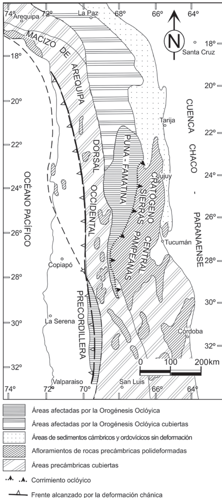
Figura 1: Mapa geológico esquemático del Cinturón Oclóyico y de su marco regional (modificado de Mon 1992). 1) Macizo de Arequipa; 2) Dorsal Occidental; 3) Precordillera; 4) Puna - Famatina; 5) Cratógeno Central (Sierras Pampeanas); 6) Cuenca Chaco - Paranaense.
