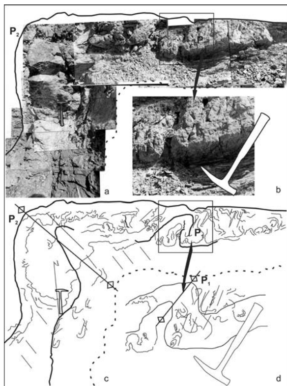
Figura 9: Detalle del afloramiento (27°42'10.2'' S - 67°57'20.5'' O). a) y b) Limolitas y volcanitas deformados según dos episodios de plegamiento superpuestos, P_1 y P_2 . c) y d) Detalle de los niveles epiclásticos plegados y el clivaje de plano axial correspondiente a P_1 .
