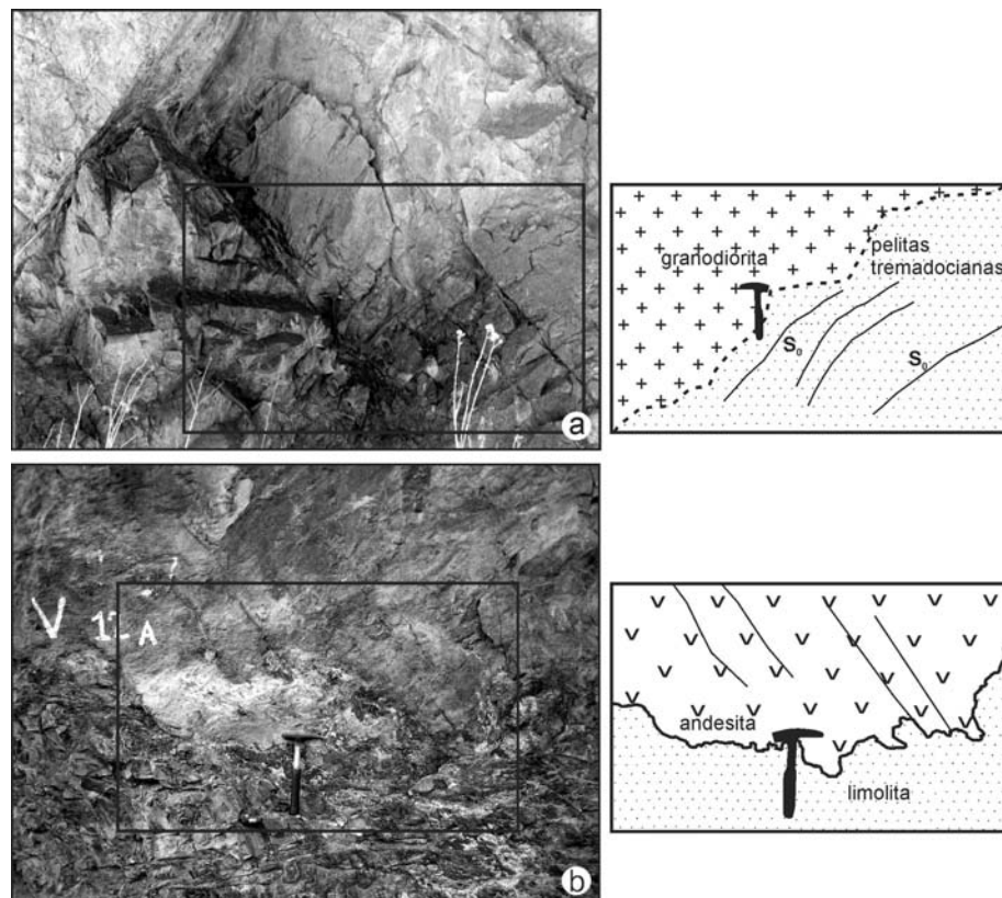
Figura 4: a) Afloramiento ( 27^\circ42'10.4'' S - 67^\circ57'05.3'' O) donde se encuentra el contacto entre la granodiorita de Las Angosturas y facies epiclásticas pelíticas con estratificación primaria ( S_0 ). A la derecha se esquematiza el contacto. b) Bancos de limolitas en contacto con niveles efusivos andesíticos. El conjunto está plegado y con desarrollo de clivaje de plano axial (ubicación del afloramiento 27^\circ42'10.4'' S - 67^\circ56'54.8'' O). Esquema de la relación a la derecha.
