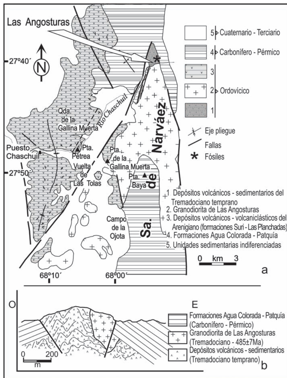
Figura 2: a) Mapa geológico del norte de la sierra de Narvárez (modificado de Cisterna 1994). b) Perfil geológico del tramo de Las Angosturas, con orientación aproximada a lo largo del paralelo de 27° 42' S.
