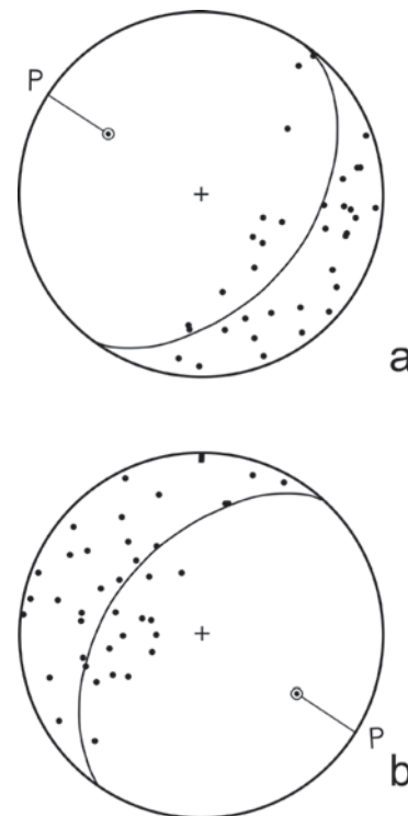
Figura 10: Datos de orientación de las estructuras medidas en el campo, graficadas en una red estereográfica equiareal. a) Plegamiento P_1 de la sucesión tremadociana temprana. b) Plegamiento P_2 medido en la misma sucesión.
