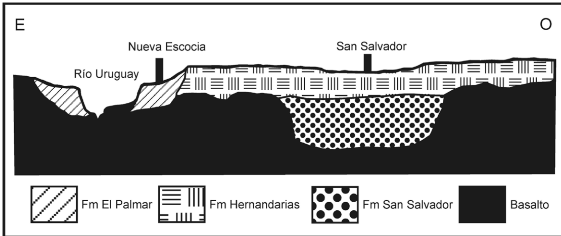
Figura 1: Perfil geológico esquemático del este de Entre Ríos a la latitud 31° 40'S (tomado y modificado de Iriondo y Kröhling 2007).
