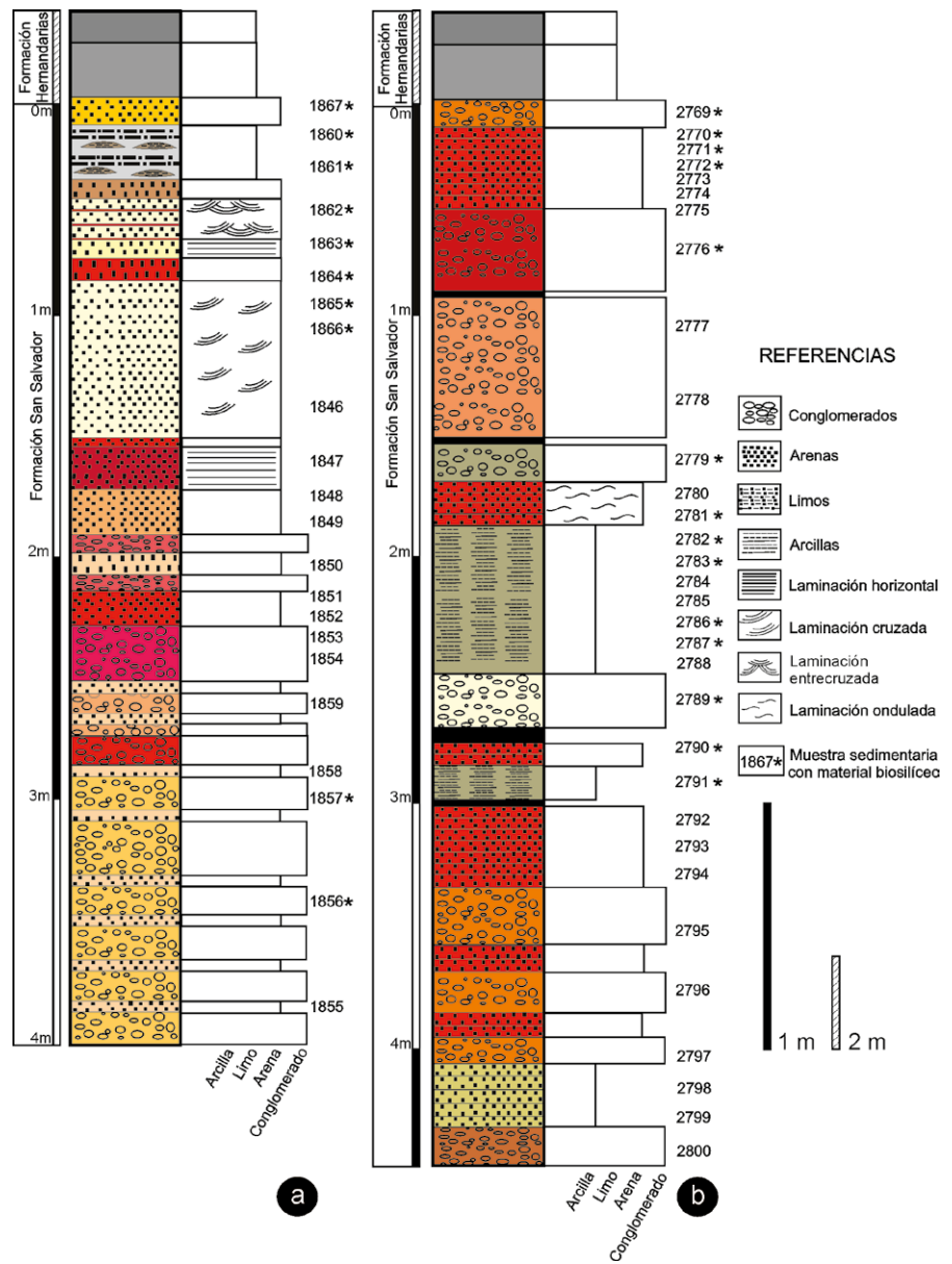
Figura 4: Perfiles sedimentológicos esquemáticos de la Formación San Salvador, a) perfil Salvia, b) perfil Concordia.
