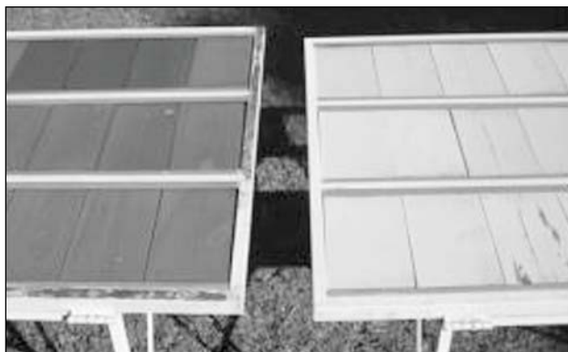
FIGURA 1. Intemperización externa.
