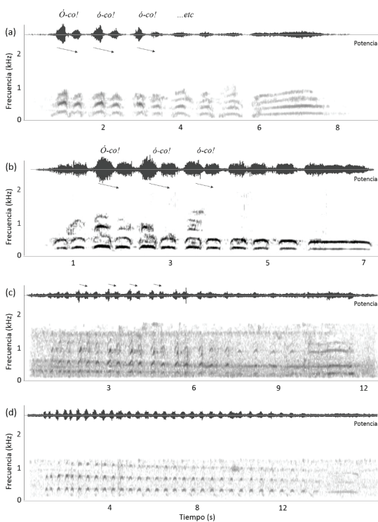
Figura 5. Audiospectrogramas de las vocalizaciones de proclamación territorial tipo B de Tigrisoma lineatum . (a) Tigrisoma lineatum marmoratum , estancia La Fidelidad, departamento Patiño, Formosa, Argentina (registro BLL421-71, registro XC300939; Xeno-canto Foundation 2015). (b) Tigrisoma lineatum marmoratum , estancia La Fidelidad, departamento Patiño, Formosa, Argentina (registro BLL421-73, registro XC300940; Xeno-canto Foundation 2015). (c) Tigrisoma lineatum marmoratum , riacho Monte Lindo, departamento Formosa, Formosa, Argentina (registro BLL438-07, registro XC300941; Xeno-canto Foundation 2015). (d) Tigrisoma lineatum lineatum , Sani Lodge, Napo, Ecuador (registro XC120559; Xeno-canto Foundation 2015).
