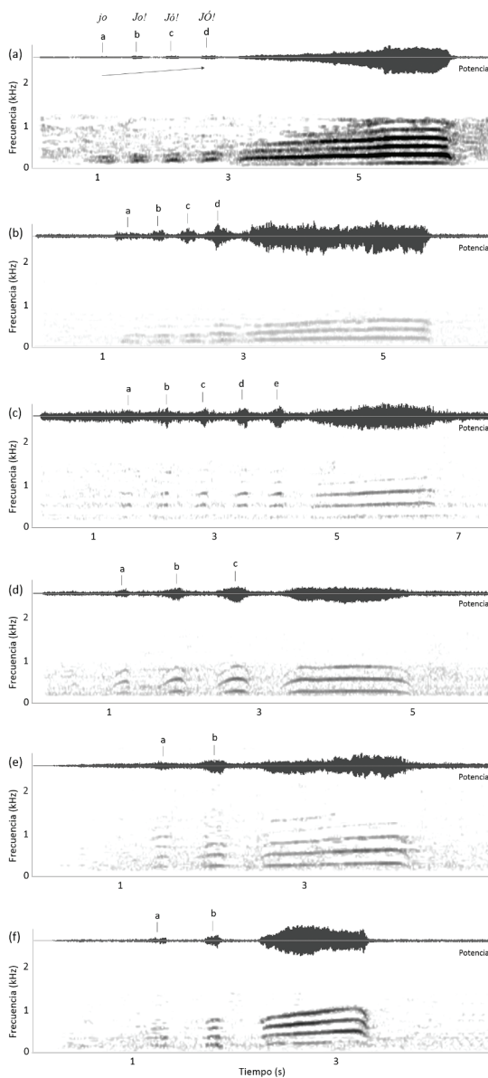
Figura 3. Audioespectrogramas de las vocalizaciones de proclamación territorial tipo A de Tigrisoma lineatum . (a) Tigrisoma lineatum marmoratum , río Pixaim (Ruta Transpantaneira), Mato Grosso, Brasil (Marantz y Zimmer 2006). (b) Tigrisoma lineatum lineatum , Resguardo Unificado Selva de Matavén, Cumaribo, Vichada, Colombia (registro XC117947; Xeno-canto Foundation 2015). (c) Tigrisoma lineatum lineatum , Cocha Juárez, Manu Lodge, Madre de Dios, Perú (registro ML184973; Cornell Lab of Ornithology 2015). (d) Tigrisoma lineatum lineatum , Campina do Vapor, Autazes, Amazonas, Brasil (Naka et al. 2008). (e) Tigrisoma lineatum lineatum , ExplorNapó y ACTS, Loreto, Perú (registro XC87242; Xeno-canto Foundation 2015). (f) Tigrisoma lineatum marmoratum , Flor d'Oro, Parque Nacional Noel Kempff Mercado, Santa Cruz, Bolivia (pista 1; Mayer 2000).
