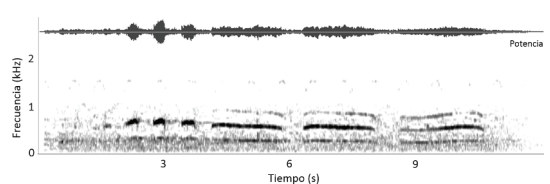
Figura 4. Audioespectrograma de la vocalización de proclamación territorial tipo A atípica de Tigrisoma lineatum registrada en el humedal de Yalare, Esmeraldas, Ecuador (registro 9; Moore et al. 2013).
