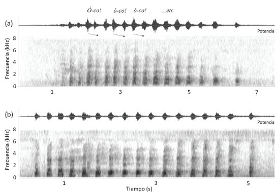
Figura 6. Audiospectrogramas de las vocalizaciones de alarma en vuelo de Tigrisoma lineatum . (a) Tigrisoma lineatum marmoratum , embalse Itiyuro, río Carapay, Tartagal, Salta (pista 1; López-Lanús 2008). (b) Tigrisoma lineatum marmoratum , cerca de Trinidad, ruta a Santa Cruz, Beni, Bolivia (pista 3; Mayer 2000).
