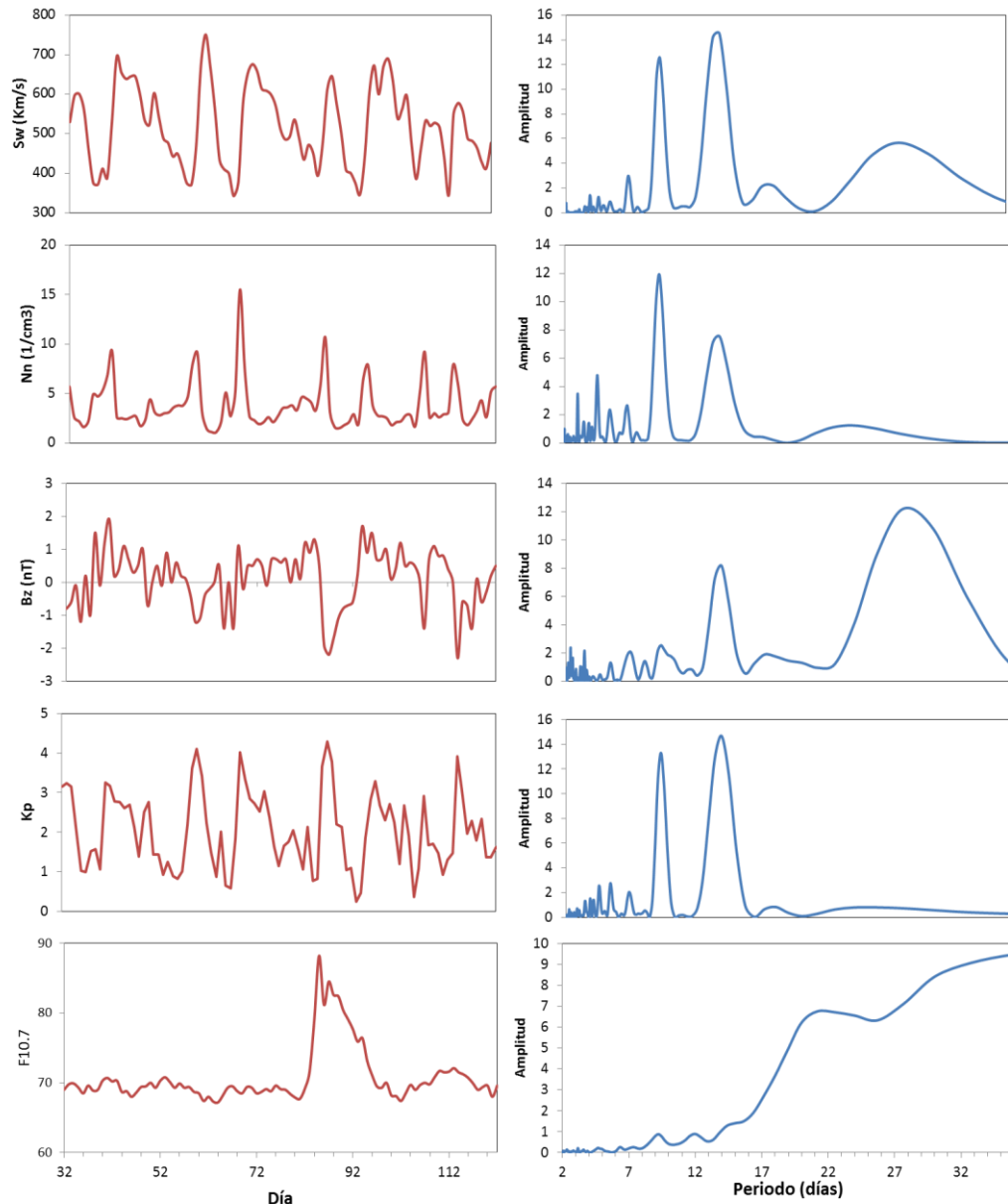
Figura N°2: Variación de la velocidad del viento solar ( Sw , Km/s), la densidad del viento solar ( Nn , cm^{-3} ), la componente Bz de IMF (nT), el índice Kp y F10.7 para el periodo comprendido entre los días 32 y 122 de 2008 (izquierda) y sus respectivos periodogramas de Lomb-Scargle (derecha).
