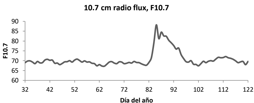
Figura N°1: índice F10.7 para el periodo comprendido entre los días 32 y 122 de 2008.
