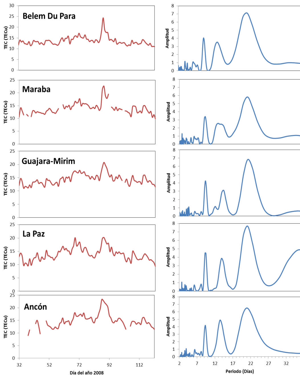
Figura N°3: Valores de TEC (izquierda) y su correspondiente periodograma de Lomb-Scargle (derecha) para las estaciones analizadas (de arriba hacia abajo): Belem Du Para, Maraba, Guajara-Mirim, La Paz y Ancón entre los días 32 y 122 de 2008.
