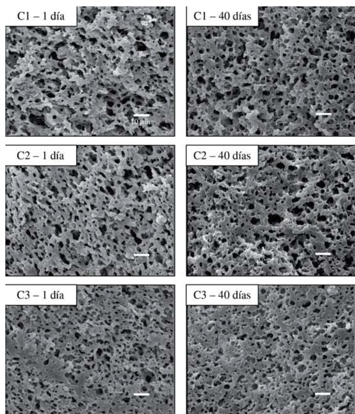
FIGURA 1 - Micrografías SEM a 1200X de las muestras a 1 y 40 días de maduración para las condiciones C1, C2 y C3. La barra blanca representa una escala de 10 \mu m.
