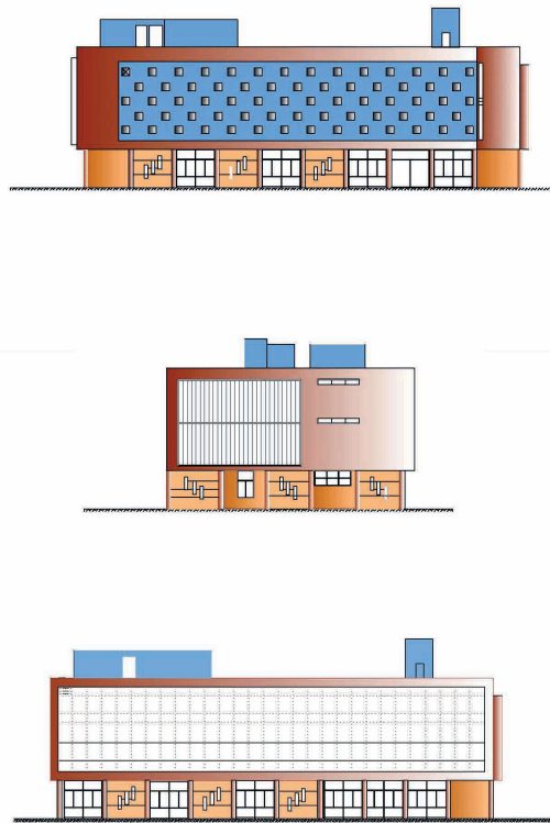
Fig.1 Fachadas del edificio de OSSE en San Juan, Argentina.
