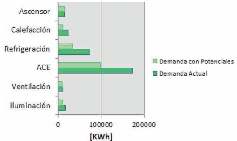
Fig.10 Comparación entre demanda eléctrica actual y demanda con potenciales de eficiencia energética aplicados en espacio de oficinas.
