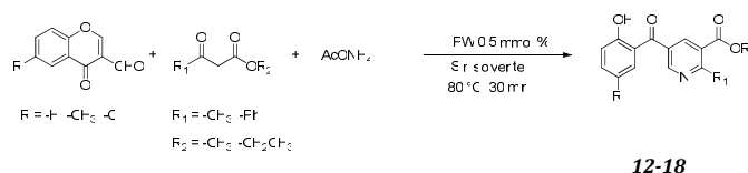
Figura 3. Reacción general para la obtención de piridinas a partir de 3-formilcromona como aldehído de partida.
