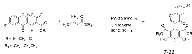
Figura 2. Última etapa en la obtención de 1,4-dihidropiridinas en varios pasos.
