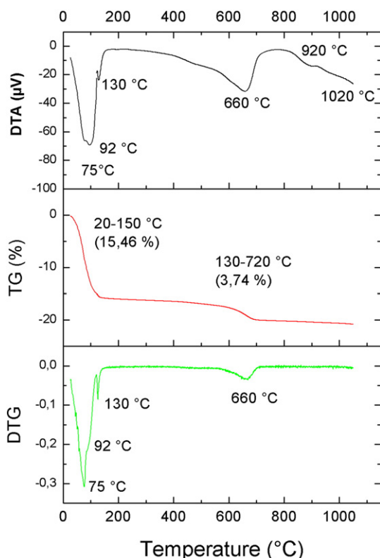
Fig. 2. Bent-0 DTA-TG-DTG analysis.
