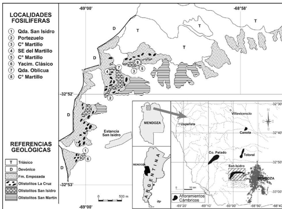
Figura 1. Mapa de ubicación de afloramientos de rocas cámbricas y de localidades fosilíferas de San Isidro, Precordillera de Mendoza, Argentina.
