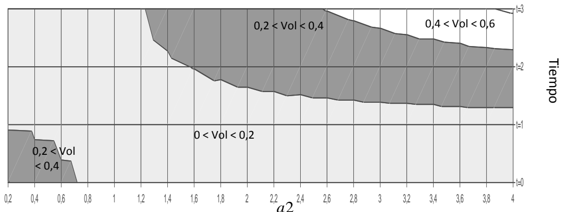
Gráfico 5: Impacto no lineal de a2 sobre la volatilidad del ciclo del empleo
