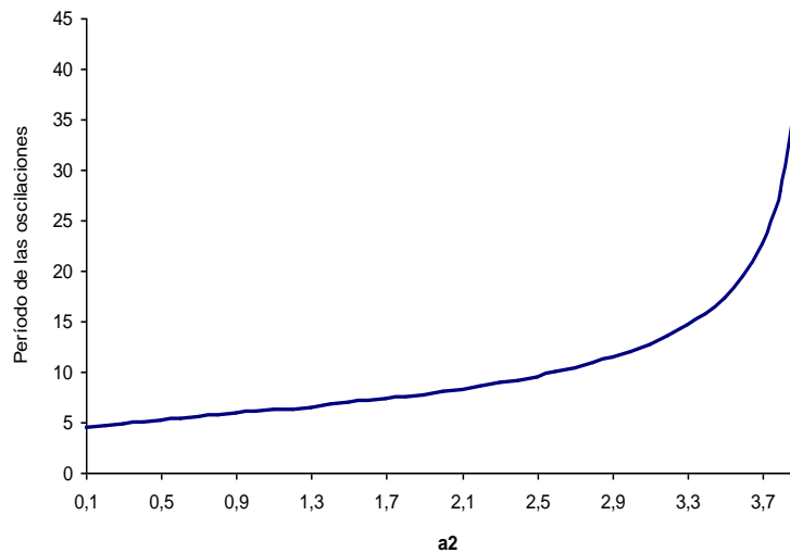
Gráfico 15: Relación entre la duración del ciclo (período de oscilación) y a2
