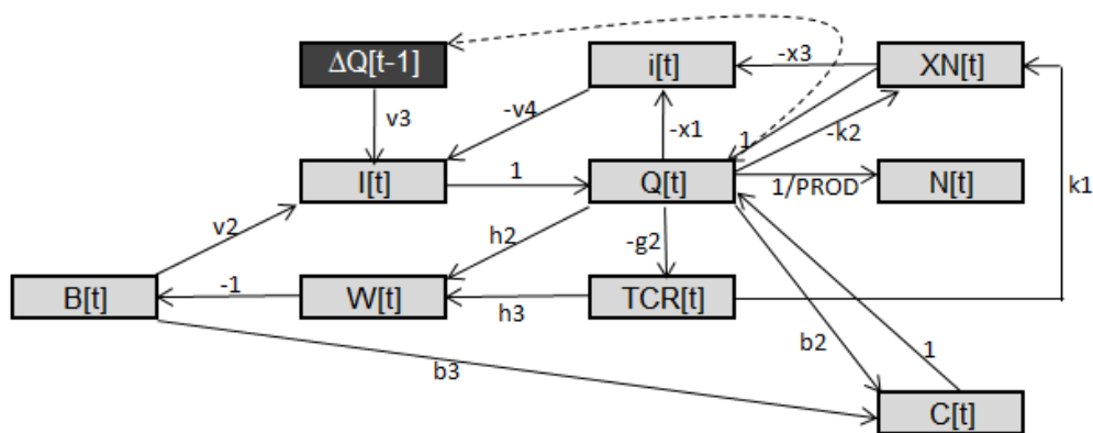
Gráfico 10: Flujograma de las ecuaciones estructurales del modelo para economía abierta, con tipo de cambio fijo y libre movilidad de capitales
