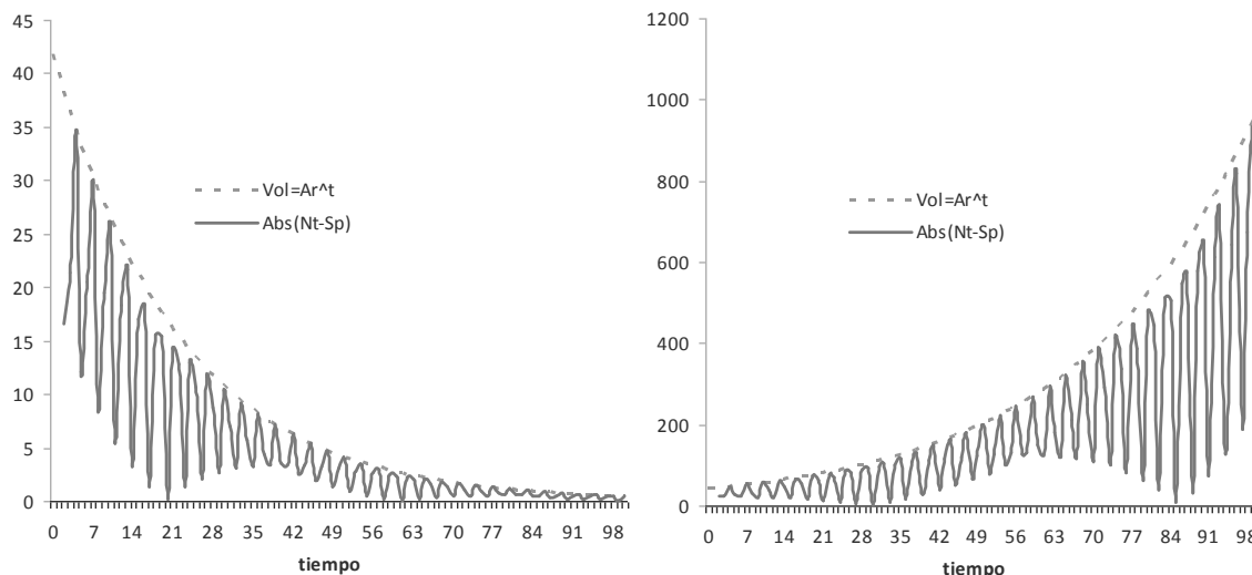
Gráfico 6: Evolución de la volatilidad del ciclo en entornos convergentes y divergentes
