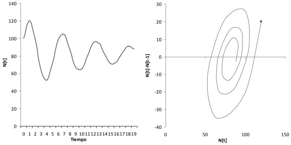
Caso 1: -0.5 < a_2 < 1 : "Oscilaciones convergentes"
