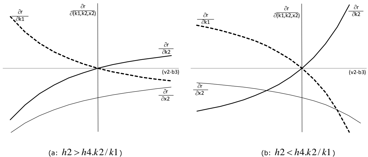
Gráfico 9: Efectos de la apertura comercial sobre la volatilidad del ciclo económico en un esquema de tipo de cambio flexible y restricciones a la movilidad de capitales
