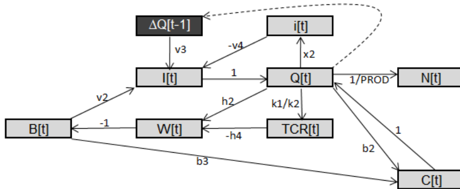
Gráfico 7: Flujograma de las ecuaciones estructurales del modelo para economía abierta, con tipo de cambio flexible y restricciones a la movilidad de capitales
