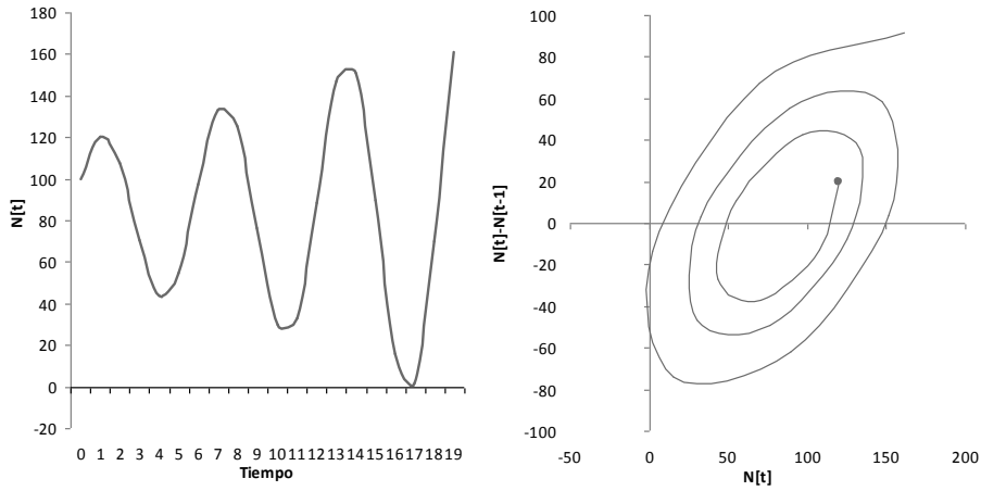
Caso 2: 1 < a_2 < 4 : "Oscilaciones divergentes"
