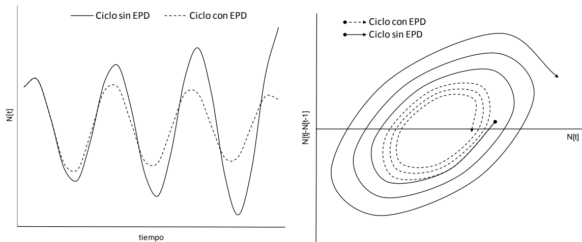
(a) Régimen de demanda de tipo wage-led
