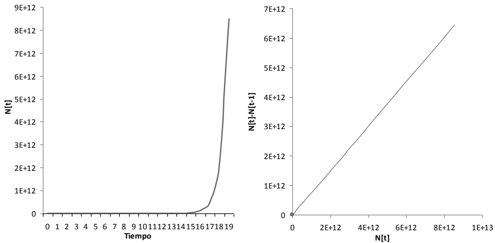
Caso 3: a_2 > 4 : "Variaciones monótonas explosivas"
