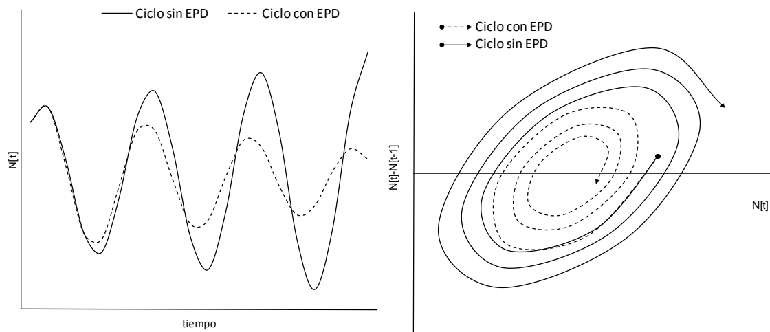
(b) Preponderancia del efecto ingreso de la EPD
