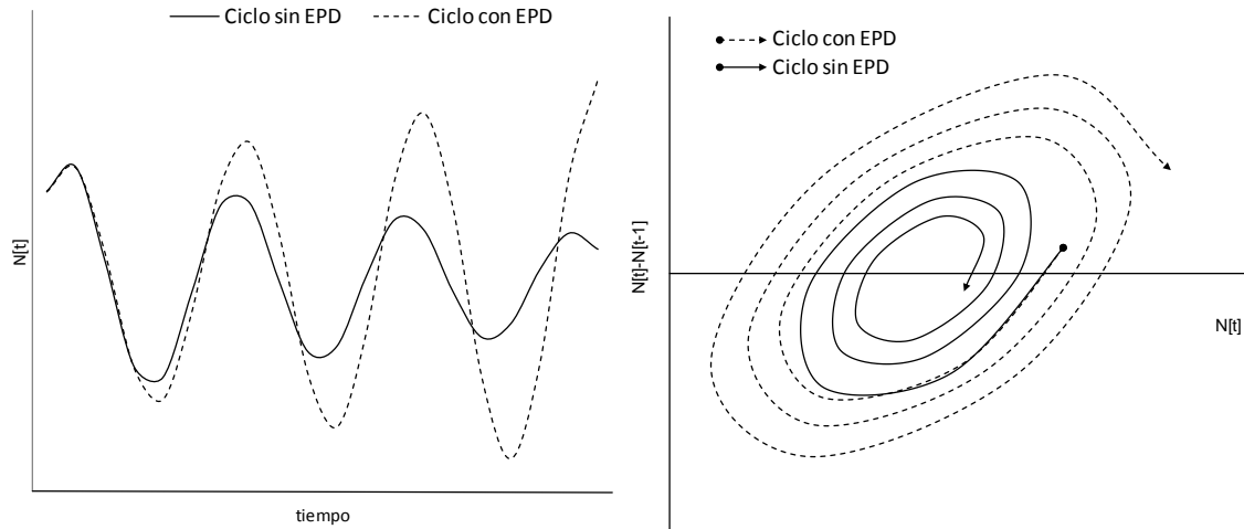
(a) Preponderancia del efecto precio de la EPD
