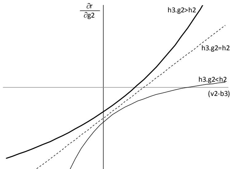
Gráfico 12: Efecto de la sensibilidad del TCR a la demanda agregada ( g_2 ) sobre la volatilidad del ciclo económico (para casos de markup procíclico, acíclico y contracíclico)
