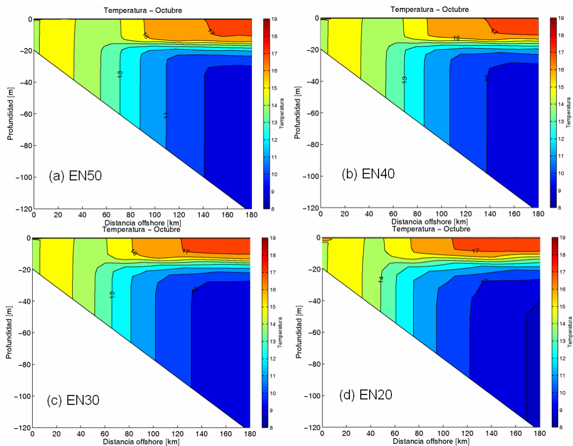
Figura 8. Corte transversal de temperatura en el mes de Octubre para el forzante y esquema de mezcla del EC para diferente número de niveles verticales. (a) 50 niveles, (b) 40 niveles, (c) 30 niveles, (d) 20 niveles.
