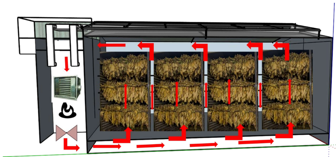
Figura 6: Diagrama de circulación de aire en el interior de la estufa durante la etapa de amarillamiento
