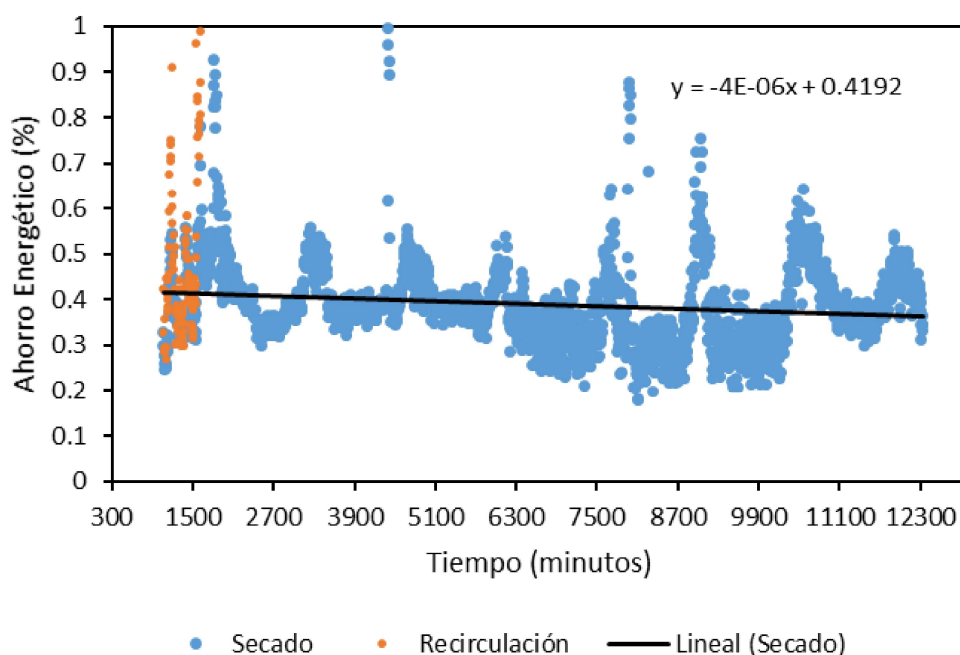
Figura 9: Ahorro calculado para la estufa intervenida
