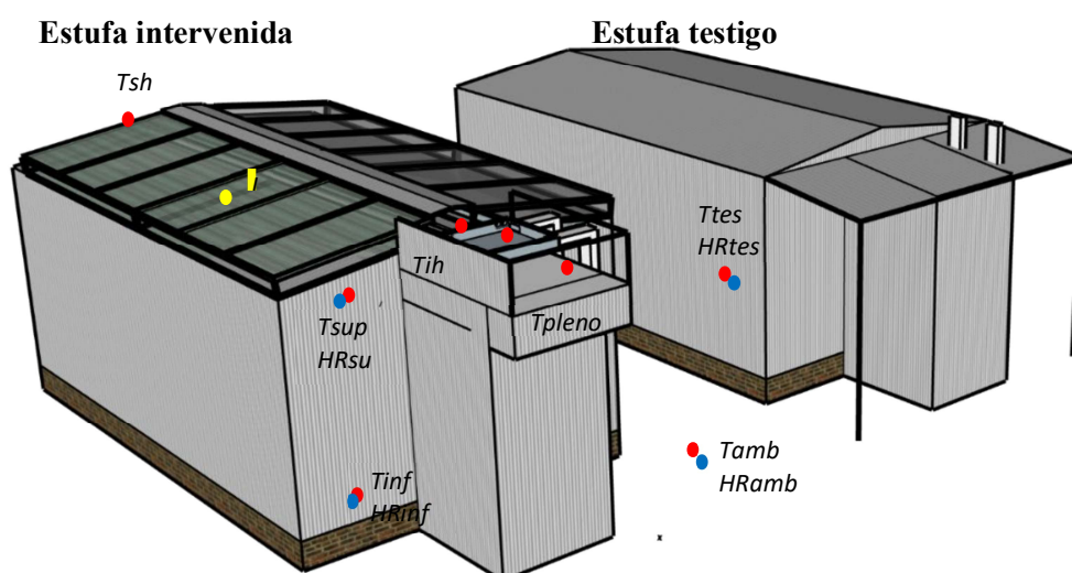
Figura 5: Esquema ubicación sensores en la estufa intervenida y su par testigo
