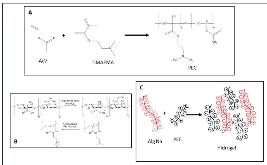
Figura 1. A) Estructura de los monómeros acetato de vinilo (AcV) y N,N-dimetilaminoetilo metacrilato (DMAEMA) para la obtención del polielectrolito catiónico (PEC). B) Estructura iónica y no iónica dependiendo del pH de los grupos carboxílicos del alginato de sodio y de la amina terciaria del DMAEMA en PEC. C) Formación del hidrogel mediante fuerza iónicas sin sonicar.
