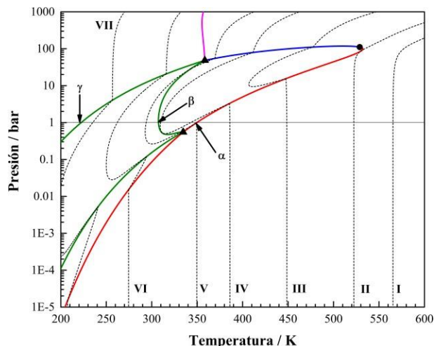
Figura 1. Proyección P versus T de una IR (EFR + E3FR + CCCs) computada para un SR en que se produce la reacción de esterificación de ácido acético (1) con etanol (2) en presencia de \text{CO}_2 (5) como inerte. \mathbf{z}^0 : fracciones molares z_1^0 = z_2^0 = 0.364 , z_3^0 = z_4^0 = 0.000 , z_5^0 = 0.272 . Curvas rojas: puntos de rocío reactivos. Curva azul: puntos de burbuja reactivos. Curva magenta: puntos de niebla reactivos. Curvas verdes: E3FR. ●: punto crítico reactivo. ▲: punto de doble saturación reactivo. Curvas de guiones negras: CsCC (asociadas) teniendo las siguientes conversiones de etanol(2): I: \chi_2 = 0.77 , II: \chi_2 = 0.79380 , III: \chi_2 = 0.84 , IV: \chi_2 = 0.8837 , V: \chi_2 = 0.91 , VI: \chi_2 = 0.94 , VII: \chi_2 = 0.99 .
