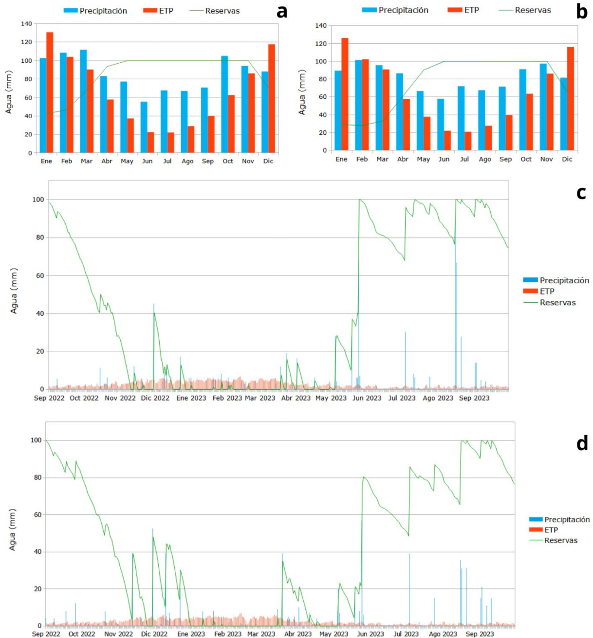
Figura 5. Balances hídricos mensuales para el período 1963-2023: a) La Plata Aero; b) Punta Indio. Balances hídricos diarios para el período septiembre 2022-septiembre 2023: c) La Plata Aero; d) Punta Indio.
