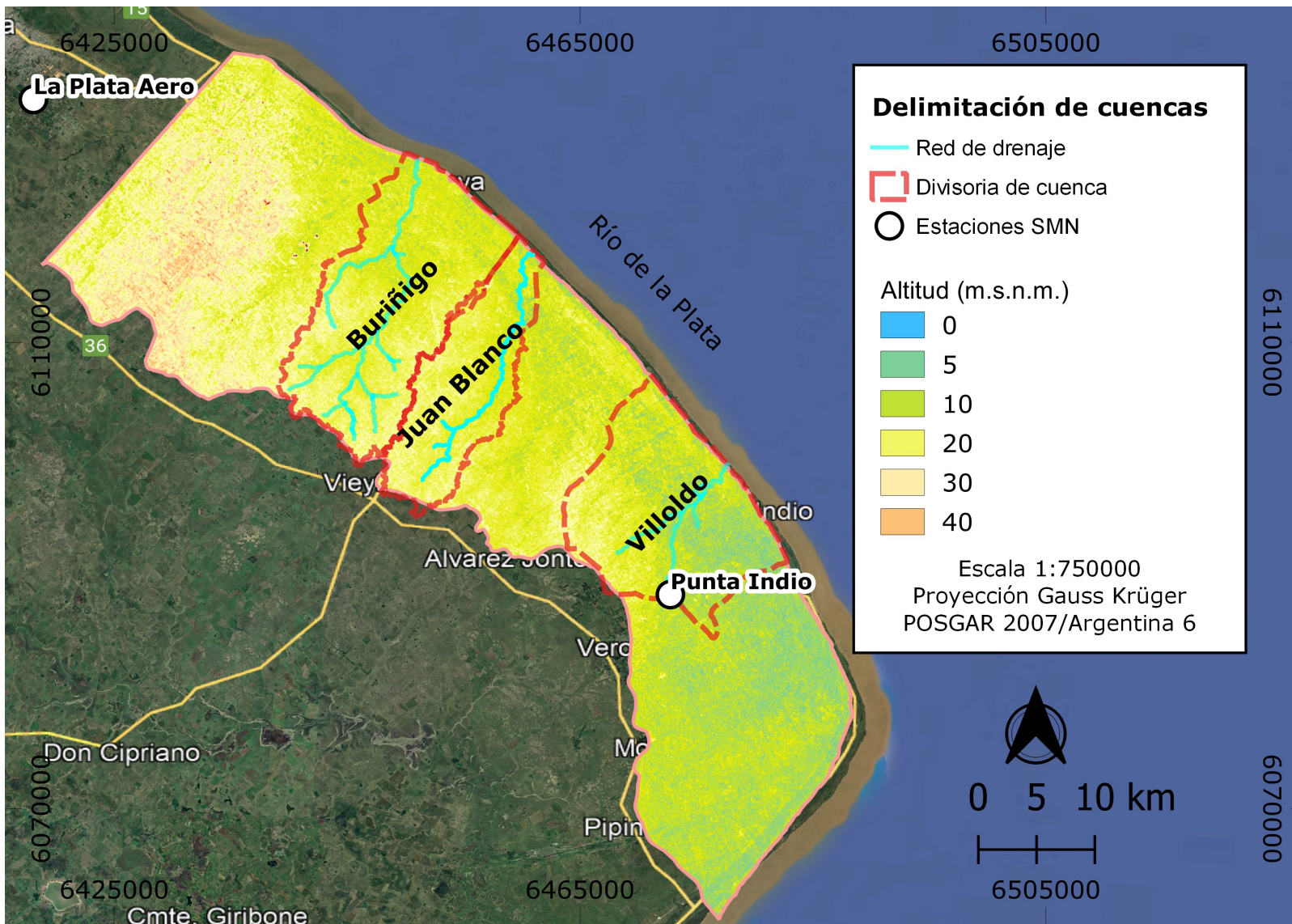
Figura 3. Delimitación de las cuencas y redes de drenaje de los arroyos estudiados, sobre MDE.
