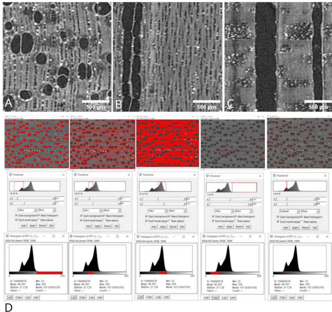
Figura 2: A-C) Láminas microtomográficas en los tres planos anatómicos -transversal, longitudinal tangencial y longitudinal radial, respectivamente- en Anacardium giganteum . Intervalos de la escala de grises que corresponden a vasos, radios, tejido fibroso, minerales y tilosis en la microtomografía de Caryocar villosum .
