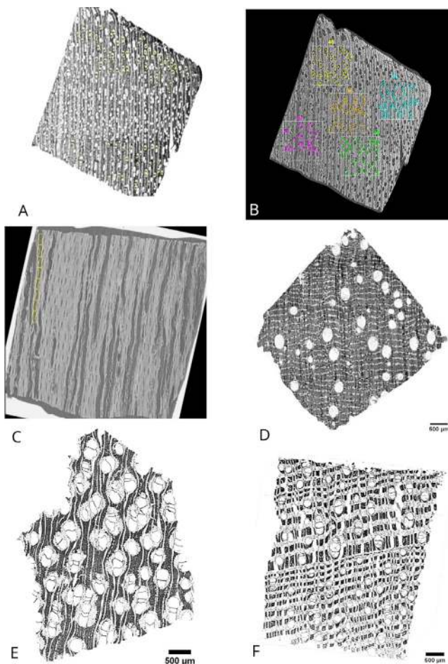
Figura 4: A) Selección de vasos para el cálculo automático del diámetro tangencial en Calycophyllum spruceanum B) Selección de vasos por área para el cálculo de la cantidad de vasos por mm 2 en Calycophyllum spruceanum ; C) Selección de vasos para el cálculo del largo de vasos en Tabebuia sp.; D) Parénquima en bandas finas observado en Licania sp; E) Parénquima paratraqueal aliforme en Diplotropis martiusii ; F) Parénquima en bandas anchas en Platanus insignis .
