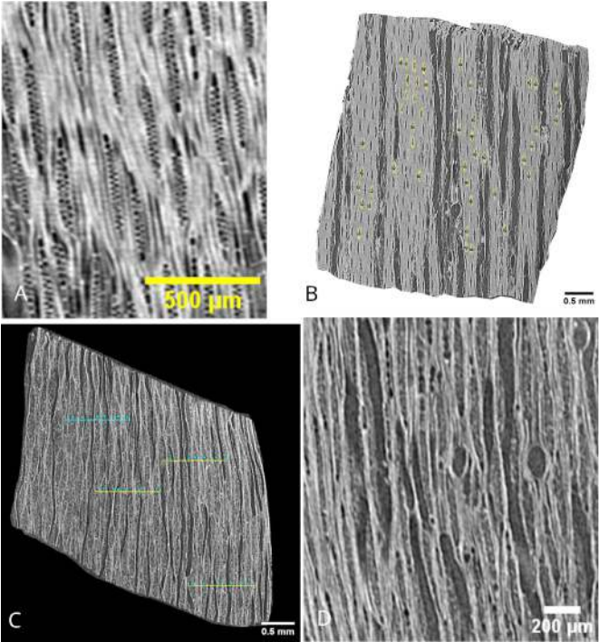
Figura 5: A) Visualización de los radios 1-3 seriados en Diplotropis martiusii ; B) Selección de los radios para cálculo de la altura de los radios en Tabebuia sp; C) Selección de los radios para conteo de la cantidad de radios por mm en Diplotropis martiusii ; D) Visualización de ductos radiales en Diplotropis martiusii .
