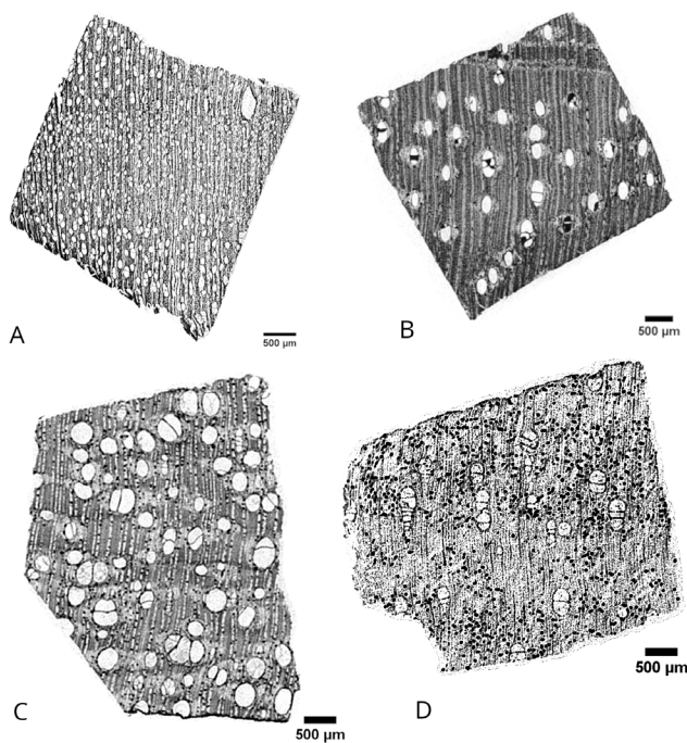
Figura 3: Anillos de crecimiento, tipo de porosidad, tipo de distribución de los vasos, presencia de depósitos en los vasos observados en A) Calycophyllum spruceanum ; B) Hymenaea sp; C) Anacardium giganteum ; D) Hura crepitans .
