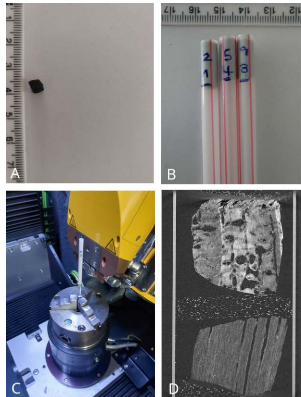
Figura 1: Preparación y montaje de las muestras para la adquisición de microtomografías. A) cubo de 4 mm de lado de carbón de madera; B) Montaje de las duplas de muestras de carbón en tubos de polipropileno; C) disposición del tubo de polipropileno con las duplas de muestras en el portaobjetos (garra) del microtomógrafo Phoenix (MZUSP); D) Corte longitudinal en una de las microtomografías de las duplas de carbones.
