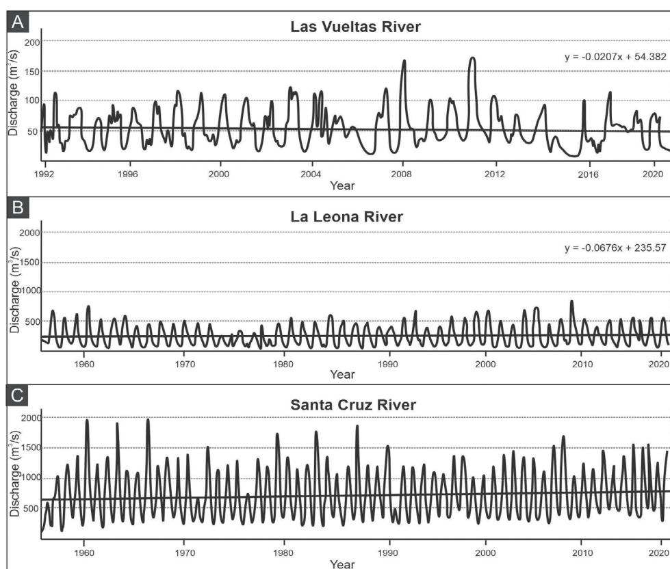
Fig. 8. A) Las Vueltas River station (interval 1991-2020). B) La Leona (interval 1956-2020). C) Santa Cruz River discharges (m³/s) at Charles Fuhr gauge station (interval 1955-2020).
