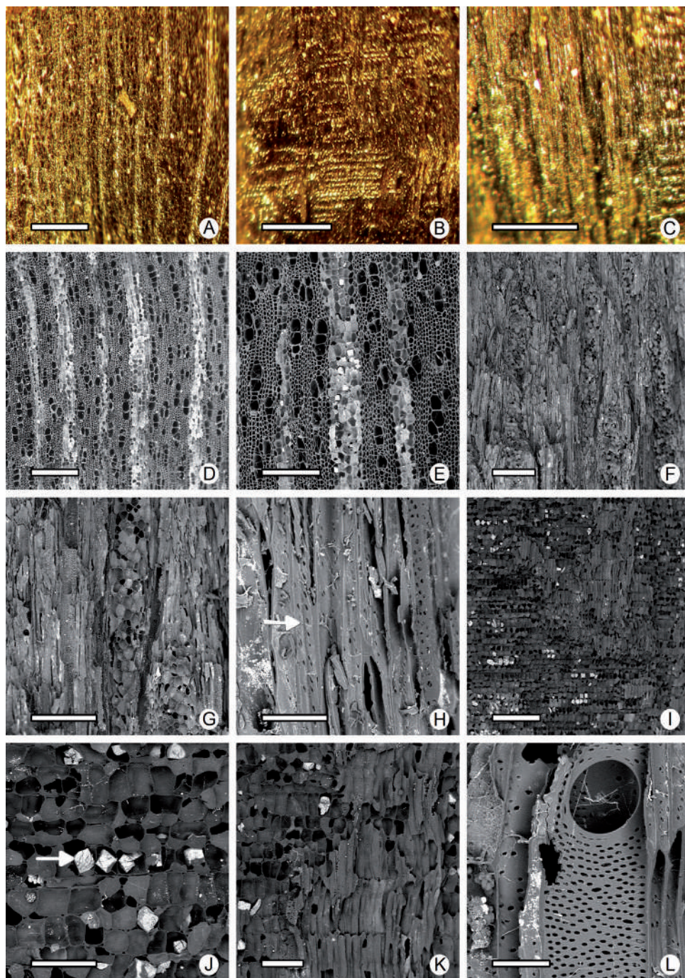
Fig. 10. Myrsine laetevirens (Mez) Arechav. (1909), CIDPALBO-MV 544, CIDPALBO-CAR 14. (A–C) en microscopio estereoscópico, (A) vista general en CT; (B) vista general en CLR; (C) vista general en CLT. (D–L) en MEB, (D) CT mostrando anillos de crecimiento demarcado y porosidad difusa; (E) detalle de vasos, parénquima, radios y fibras CT; (F) CLT mostrando radios y fibras; (G) detalle de radio multiseriado alto y ancho; (H) fibras con punteaduras pequeñas y simples; (I) vista general CLR; (J) detalle de células del parénquima radial y cristales prismáticos (flecha) CLR; (K) detalle del parénquima septado y estratificado en CLR; (L) vaso con punteaduras intervasculares alternas a subpuestas y placa de perforación simple. Escalas = 500 (A–B), 300 (D, F, I), 250 (C), 200 (E, G), 100 (J–K), 30 (H, L) \mu\text{m} .
