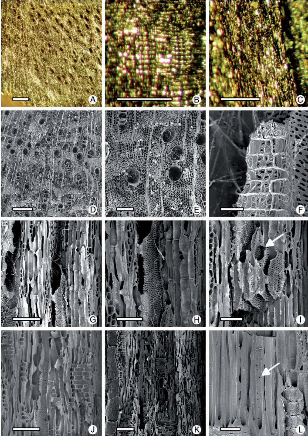
Fig. 5. Pseudalbizzia inundata (Mart.) E. J. M. Koenen & Duno (2022), CIDPALBO-MV 542, CIDPALBO-CAR 12. (A-C) en microscopio estereoscópico. (A) vista general en CT. (B) vista general en CLR. (C) vista general en CLR. (D-L) en MEB, (D) porosidad difusa en CT; (E) detalle de vasos, fibras y parénquima en CT; (F) punteaduras radio-vasculares; (G) Radios, vasos, parénquima y fibras en CLT; (H) vasos con punteaduras intervasculares alternas y parénquima septado y estratificado en CLT; (I) vaso con placa de perforación simple en CLT (flecha); (J-K) radios homocelulares en CLR; (L) detalle de fibras con punteaduras simples en CLR (flecha). Escalas = 1 (A) mm, 500 (B), 300 (D) 250 (C), 100 (E, K), 80 (G, J), 50 (H-I), 30 (L), 20 (F) \mu\text{m} .
