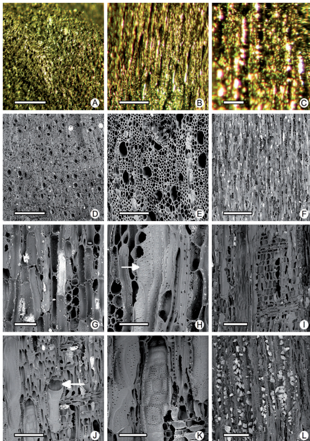
Fig. 9. Eugenia myrcianthes Nied. (1893), CIDPALBO-MV 545, CIDPALBO-CAR 15. (A-C) en microscopio estereoscópico, (A) vista general en CT; (B) vista general en CLT; (C) vista general en CLR. (D-L) en MEB, (D) porosidad difusa en CT; (E) detalle de los vasos en CT; (F) vista general en CLT; (G) detalle de parénquima septado, fibra septada y radio en CLT; (H) punteaduras intervasculares alternas y ornadas (flecha) en CLT; (I) vista general en CLR; (J) placa de perforación simple (flecha) en CLT; (K) punteaduras radio-vasculares; (L) parénquima cristalífero. Escalas = 500 (B), 300 (D), 200 (F), 100 (E, I-J), 80 (K), 50 (L), 30 (G-H) \mu\text{m} , 1 mm (A, C).
