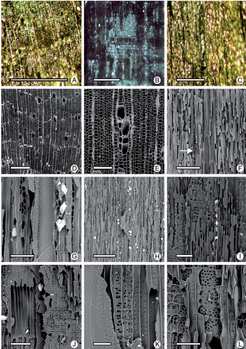
Fig. 3. Croton urucurana Baill. (1864), CIDPALBO-MV 537, CIDPALBO-CAR 7. (A) CT en microscopio estereoscópico. (B) CLR en microscopio invertido. (C) CLT en microscopio estereoscópico. (D-L) en MEB, (D) CT mostrando porosidad difusa; (E) detalle de un vaso agrupado; (F) radios uni, bi y triseriado (flecha) en CLT; (G) detalle de punteaduras intervasculares y cristales en parénquima septado en CLT; (H) vista general en CLT; (I) vista general en CLR; (J) radio, fibra y vaso con placa de perforación simple (flecha) en CLR; (K) parénquima septado y fibras con punteaduras simples; (L) punteaduras radio-vasculares. Escalas = 300 (D, H), 250 (A-C), 200 (F), 100 (E, I), 80 (G, J), 50 (L), 30 (K) \mu\text{m} .
