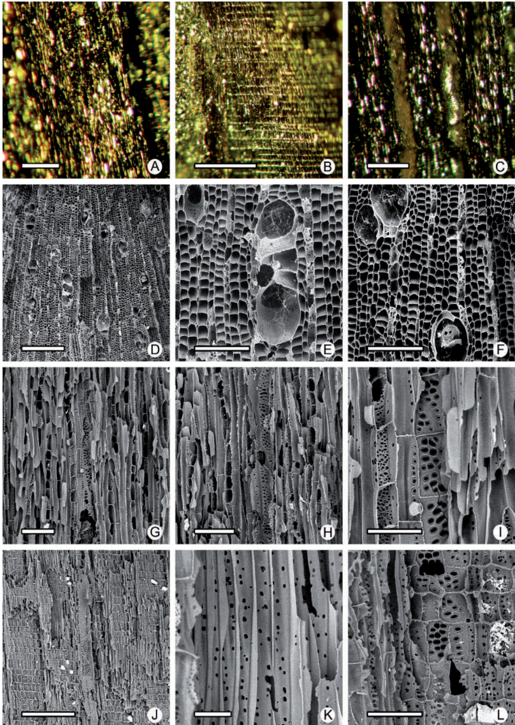
Fig. 4. Sapium haemospermum Müll. Arg., (1865) CAMPALBO-MV 543, CIDPALBO-CAR 13. (A-C) en microscopio estereoscópico; (A) vista general en CT; (B) vista general en CLR; (C) vista general en CLT. (D-L) en MEB, (D) porosidad difusa en CT; (E) detalle de un vaso en CT; (F) fibras ordenadas radialmente en CT; (G) radios mayormente uniseriados en CLT; (H) radios, fibras, parénquima y vaso en CLT; (I) detalle de vaso, parénquima y fibra en CLT; (J) vista general en CLR; (K) detalle de punteaduras en fibras en CLR; (L) punteaduras radio-vasculares. Escalas = 500 (A, B), 300 (D), 250 (C), 200 (J), 100 (E-H), 50 (I, L), 30 (K) \mu\text{m} .
