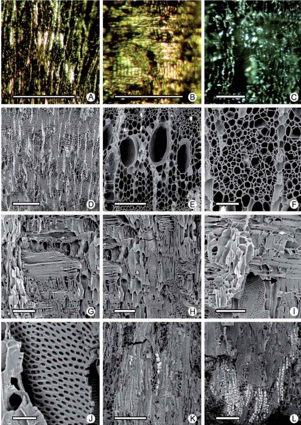
Fig. 7. Vachellia caven (Molina) Seigler & Ebinger (2006), CIDPALBO-MV 539, CIDPALBO-CAR 9. (A) CT en microscopio estereoscópico. (B) CLR en microscopio estereoscópico. (C) CLT en microscopio invertido. (D–L) en MEB, (D) vista en general en CT; (E) detalle de vasos y parénquima en CT; (F) detalle de fibras en CT; (G) vista general de CLR mostrando radios formados por células procumbentes; (H) vaso, parénquima y radio en sección longitudinal radial; (I) punteaduras intervasculares (flecha) y radio-vasculares (flecha negra) en CLR; (J) detalle de las punteaduras intervasculares alternas y ornadas; (K) vista general del CLT mostrando radios, parénquima, fibras y cristales romboidales; (L) cristales romboidales en células del parénquima axial y fibras. Escalas = 500 (A–B), 300 (D), 250 (C), 200 (J), 100 (E, G–H, K, L), 80 (I), 50 (F), 20 (J) \mu\text{m} .
