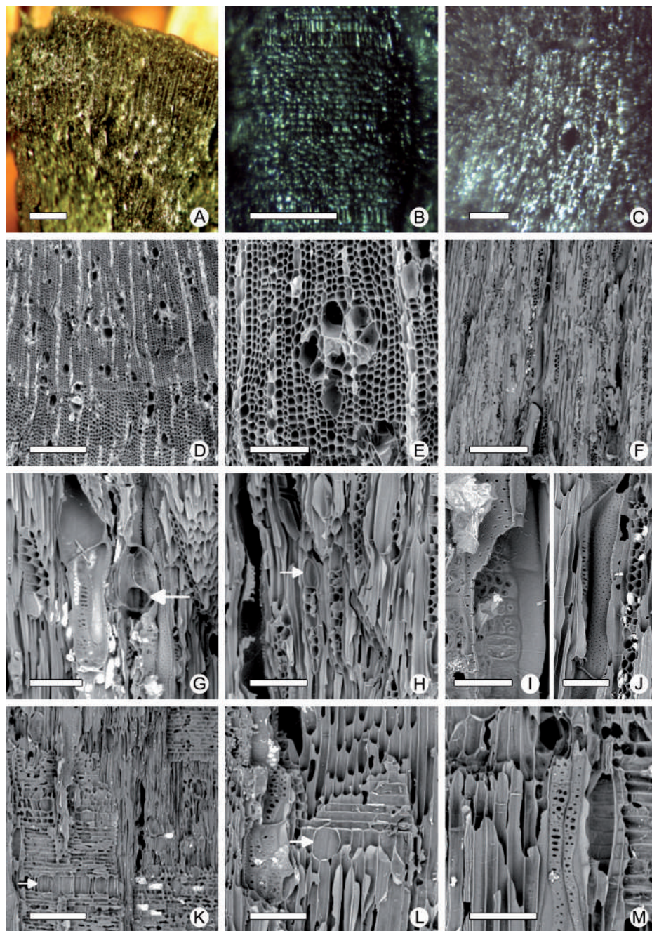
Fig. 8. Nectandra angustifolia (Schrud.) Nees & Mart. (1833), CIDPALBO-MV 538, CIDPALBO-CAR 8. (A) CT en microscopio estereoscópico. (B) CLR en microscopio invertido. (C) CLT en microscopio invertido. (D-M) en MEB, (D) vista en general en CT mostrando anillo de crecimiento y porosidad difusa; (E) detalle de vaso agrupado y fibras ordenadas radialmente en CT; (F) vista general en CLT mostrando radios, vasos y fibras; (G) vasos con tabiques oblicuos (flecha negra) y placa de perforación simple (flecha blanca); (H) CLT mostrando radios uni, bi y triseriados con células oleíferas y/o mucilaginosas (flecha); (I) punteaduras radio-vasculares; (J) punteaduras intervasculares alternas; (K) vista general CLR mostrando radios formados por células procumbentes, erectas marginales y presencia de células oleífera y/o mucilaginosas (flecha). (L) detalles de célula oleífera y/o mucilaginosa (flecha) en CLR; (M) fibras septadas y con punteaduras simples en CLR. Escalas = 300 (C-D, F), 250 (B), 100 (E, G-H, J, L), 10 (E-F) \mu\text{m} , 1 mm (A).
