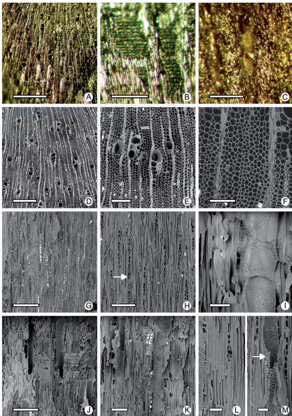
Fig. 6. Inga sp., CIDPALBO-MV 541, CIDPALBO-CAR 11. (A–C) en microscopio estereoscópico, (A) vista general en CT; (B) vista general en CLR; (C) vista general en CLT. (D–M) en MEB, (D) porosidad difusa en CT; (E) detalle de vasos, parénquima y fibra en CT; (F) detalle de las fibras sin orden aparente en CT; (G) vista general en CLT mostrando radios, fibras y parénquima cristalífero; (H) radios uni-triseriados (flecha); (I) vasos cortos con punteaduras intervasculares alternas y ornadas; (J) vista general del CLR; (K) detalle de radios, vaso, fibras y parénquima en CLR; (L) fibras septadas; (M) punteaduras radio-vasculares (flecha). Escalas = 500 (A, C), 300 (D), 250 (B), 200 (G, J), 100 (E, H, K), 50 (F, I, L), 30 (M) \mu m.
