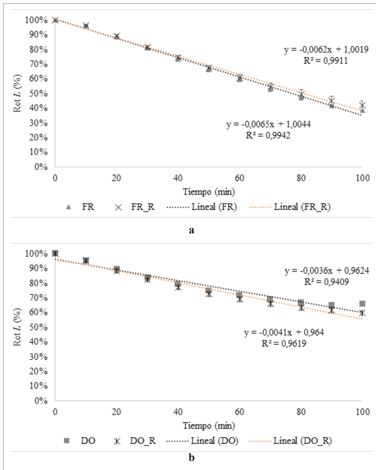
Figura 3. Retención de semi-espesor L durante el secado con MW de láminas de frutillas FR y DO, con y sin recubrimiento. a) FR+MW y FR_R+MW, b) DO+MW y DO_R+MW
