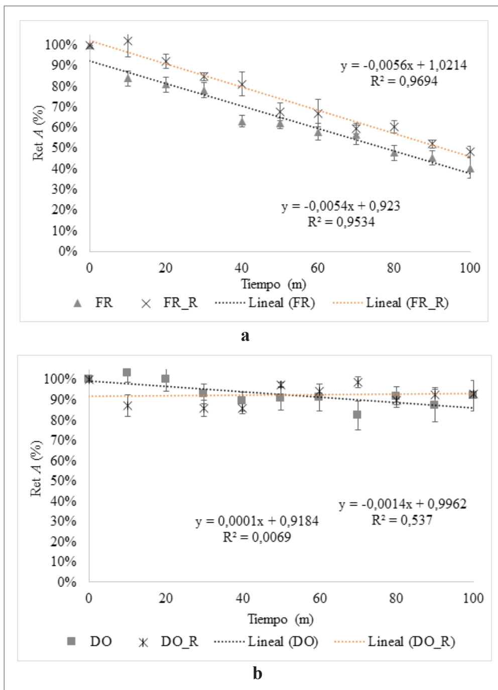
Figura 5. Retención de área (A) durante el secado con MW de láminas de fresas FR y DO, con y sin recubrimiento. a) FR+MW y FR_R+MW, b) DO+MW y DO_R+MW
