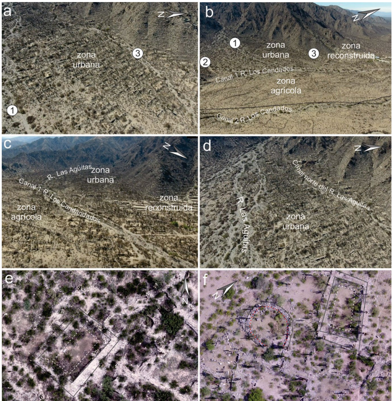
Figura 3. (a) vista de la zona urbana del asentamiento: (1) canal del río Las Agüitas, (3) canal norte del río Las Agüitas; (b) vista del encuentro entre los abanicos aluviales de Las Agüitas y Los Candados junto con los sectores del sitio, (2) canal sur río Las Agüitas; (c) septentrional de la zona agrícola y el encuentro de pendientes con el canal trezado del río Los Candados tras la confluencia con Las Agüitas; (d) zona urbana
