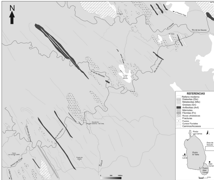
Figura 2. Mapa litológico del sector centro-oriental de la sierra de Comechingones.
