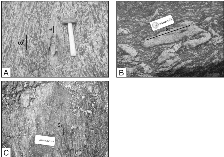
Figura 5. Foliaciones metamórficas. A) Fotografía de campo de resistor gnéusico incluido en la unidad metatexítica, se ha señalado la foliación relicta (S 1 ) la cual actualmente está reorientada en igual sentido que la foliación regional (S 2 ). Masa = 300 mm. B) Metatexita con leucosoma plegado y estirado, se indica el sentido de la foliación S 2 . Escala = 50 mm. C) Foto de campo donde se observa la foliación milonítica S 3 dada por la alternancia de folias ricas en Chl y Ser. Escala = 50 mm.
