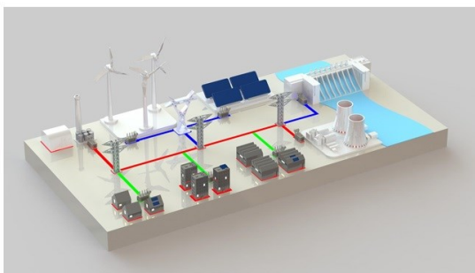
Imagen 3 | Izquierda: diseño por computadora del escenario 8 . Derecha: implementación real del escenario 8 . Fuente: elaboración propia
