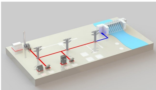
Imagen 2 | Izquierda: diseño por computadora del escenario 2 . Derecha: implementación real del escenario 2 . Fuente: elaboración propia
