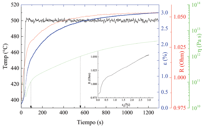
Figura 4. Comportamiento de \epsilon , R , y \eta en un ensayo con \sigma = 25 MPa. Gráfico inserto: relación R(\epsilon) .
