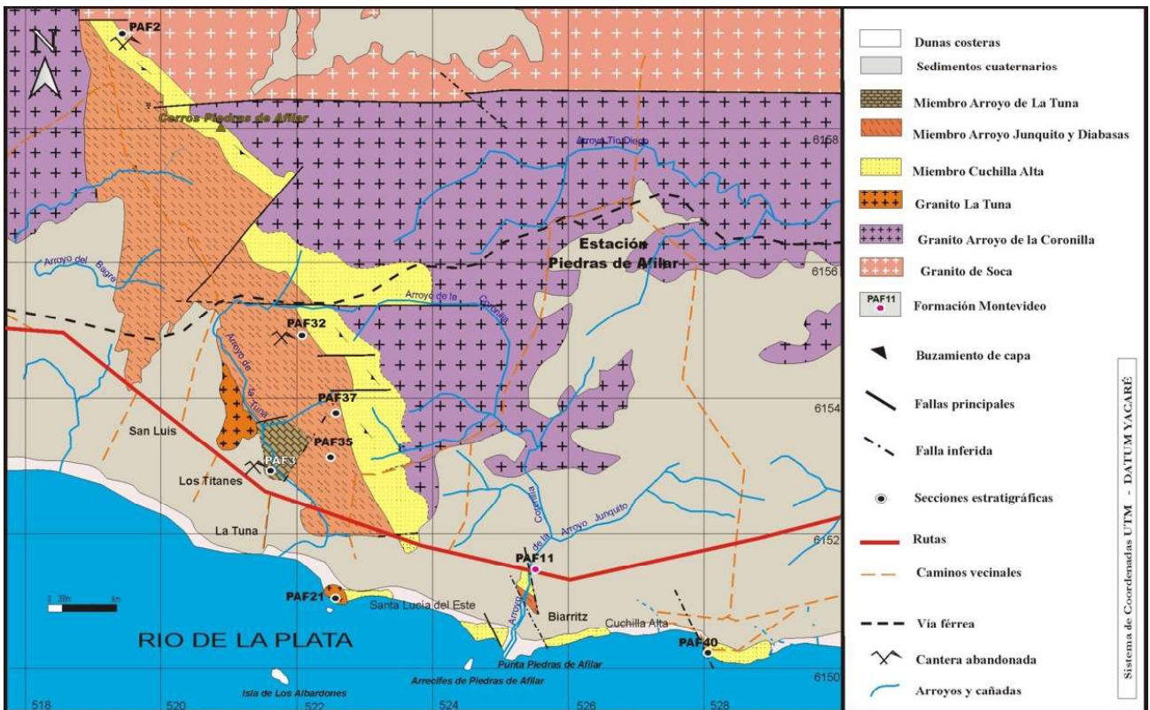
FIGURA No.2: Mapa geológico de la zona Cuchilla Alta-Piedras de Afilar, Departamento de Canelones, Uruguay (Coordenadas UTM, Datum Yacaré). Principales secciones estratigráficas: PAF2: perfil tipo del MCA; PAF 3: perfil tipo del MAT; PAF 35: perfil tipo del MAJ. Zonas de afloramiento relevantes: PAF 21: Araminda; PAF 40: areniscas de Cuchilla Alta
