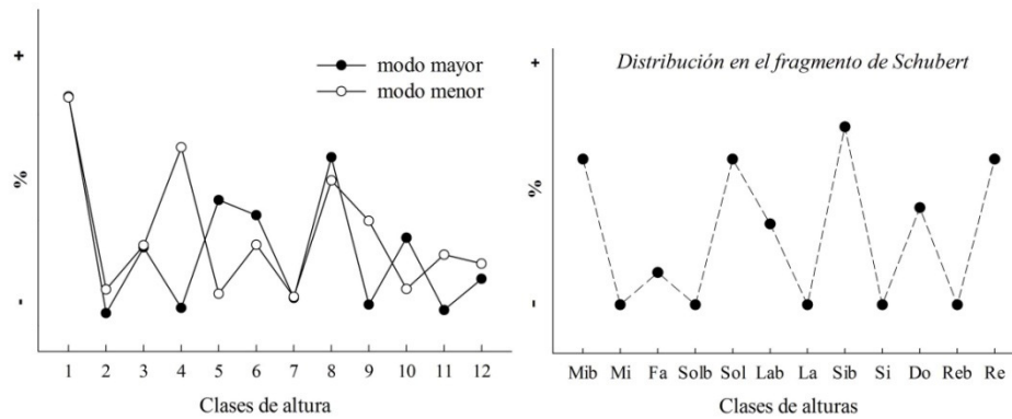
Figura 2. Izquierda: distribuciones de clases de altura típicas de piezas Tonales (después de Krumhansl, 1990); 1= tónica. Derecha: distribución en los fragmentos de la Figura 1.
