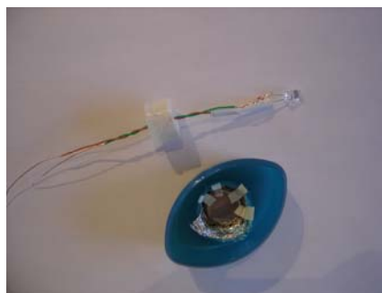
Fig. 2. Circuito del led, cables y la pila.
