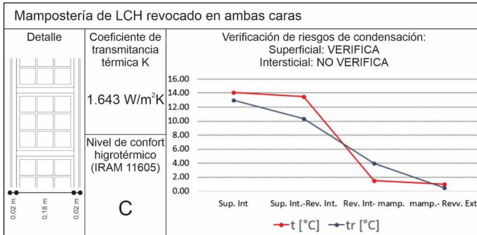
Figura 2. Comportamiento higrotérmico del cerramiento vertical exterior Elaboración propia
