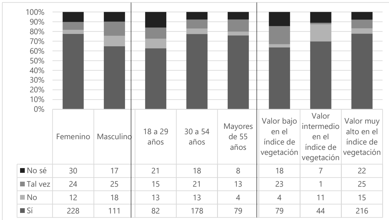
Figura 3. ¿Le parece que este espacio tiene una función importante para dar respuesta a los impactos del cambio climático? Distribución de las respuestas según género y edad de los encuestados y vegetación en el EVP donde se realizó la encuesta.
